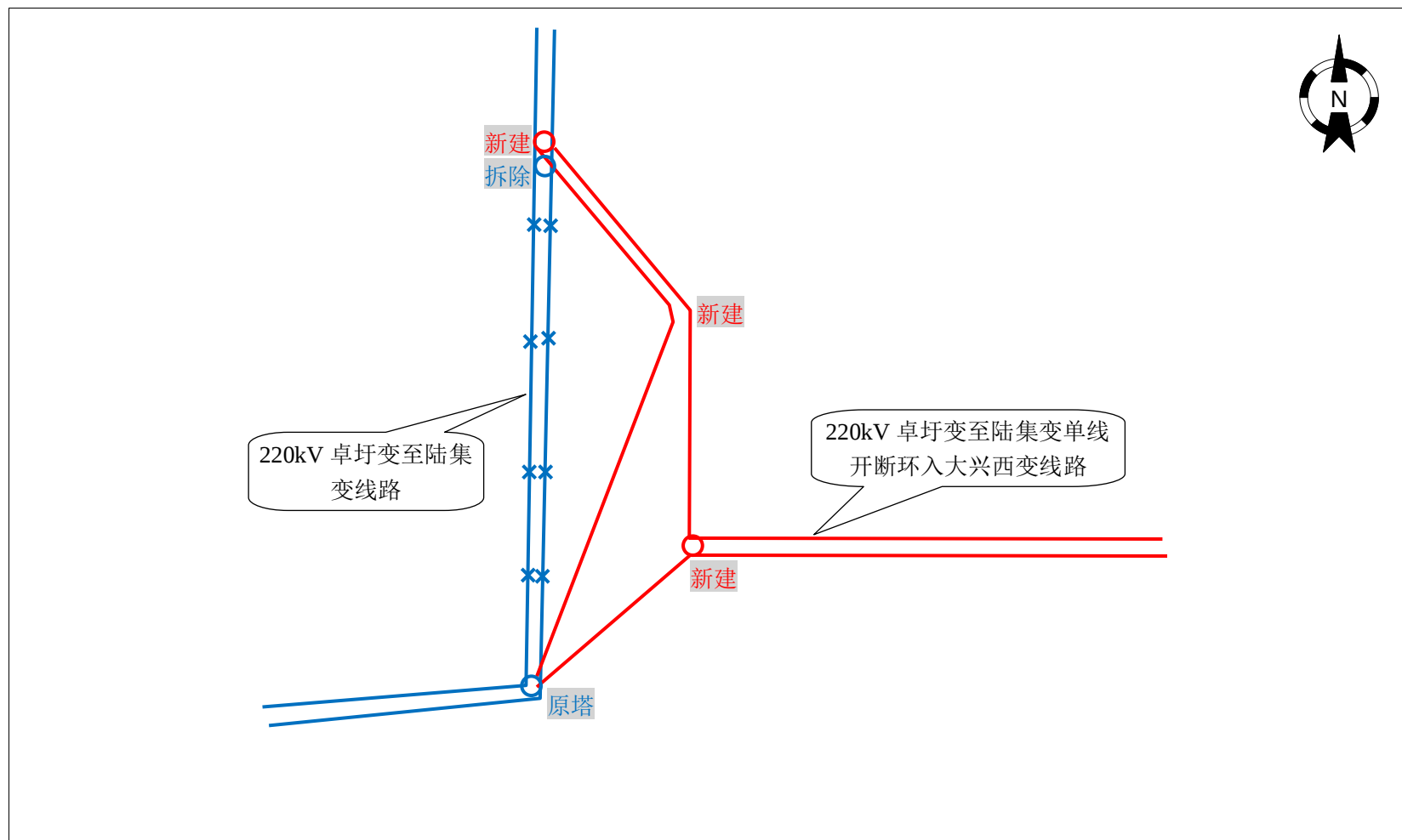
附图 2 220kV 卓圩变至陆集变单线开断环入大兴西变线路开环示意图 (b)
