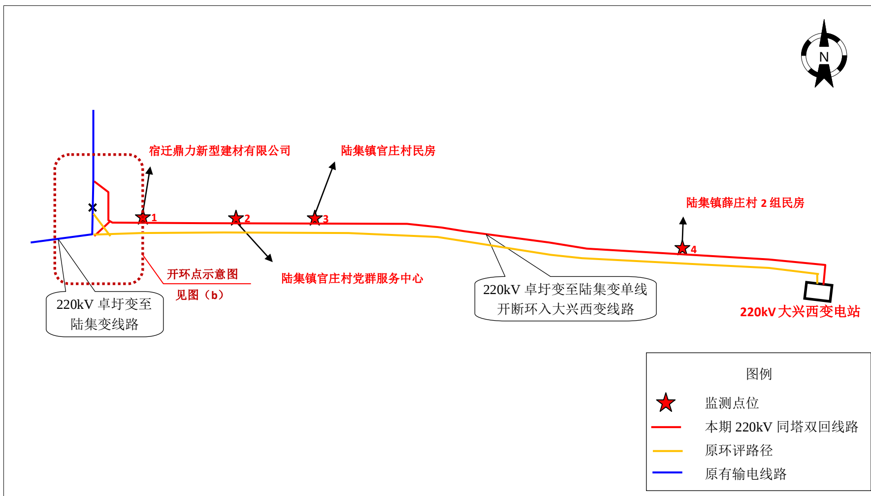
附图 2 220kV 卓圩变至陆集变单线开断环入大兴西变线路路径及监测点位示意图 (a)
