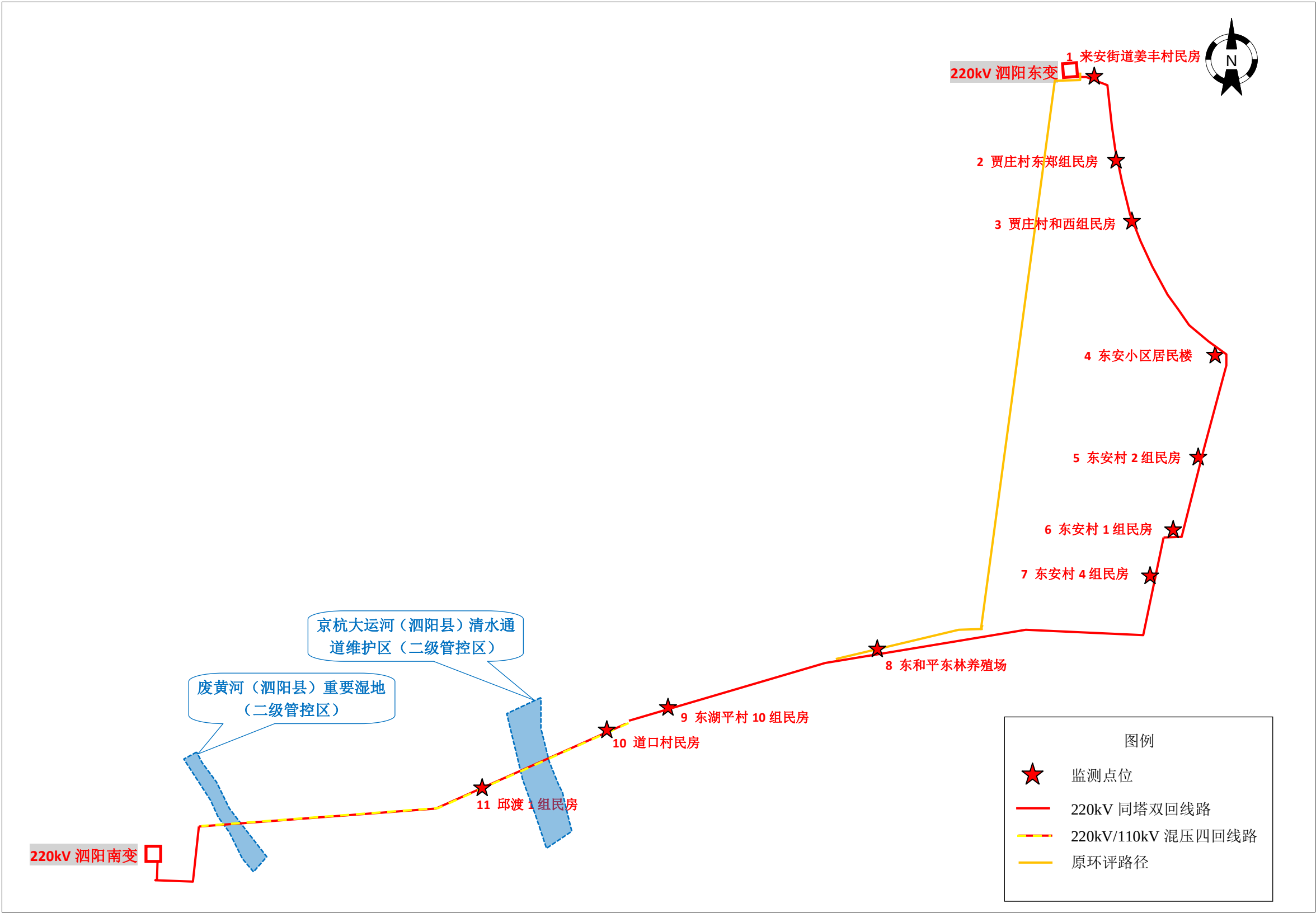
附图 2 220kV 泗阳南至泗阳东线路路径及监测点位示意图
