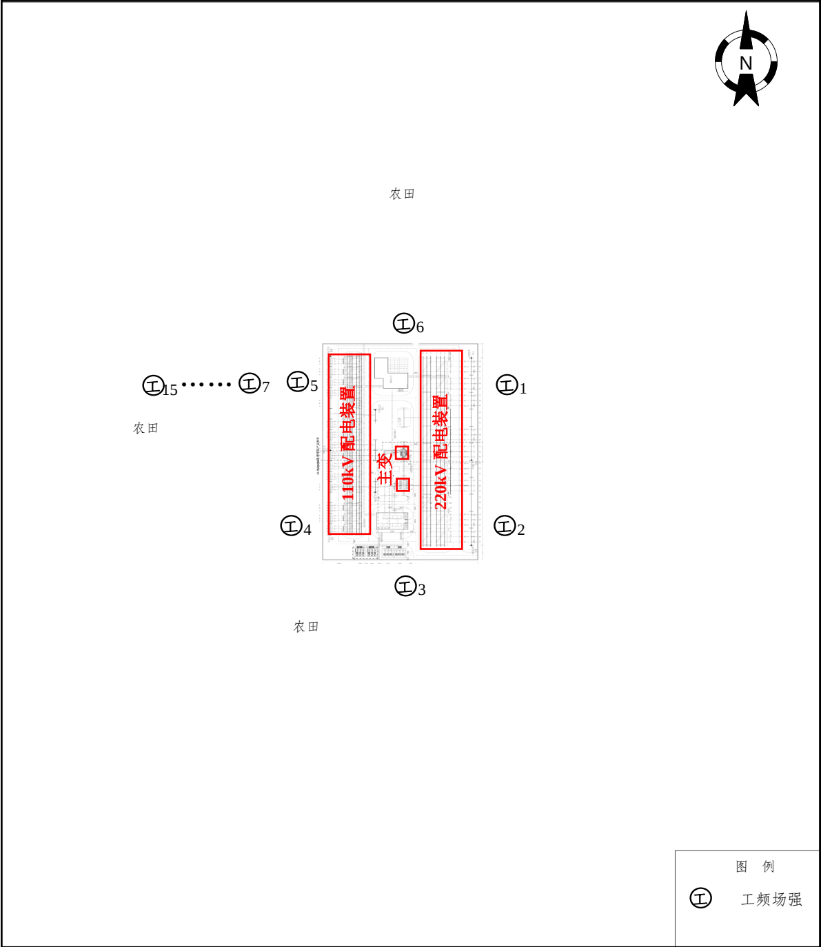
附图 4 220kV 北塘变电站（类比站）监测点位示意图
