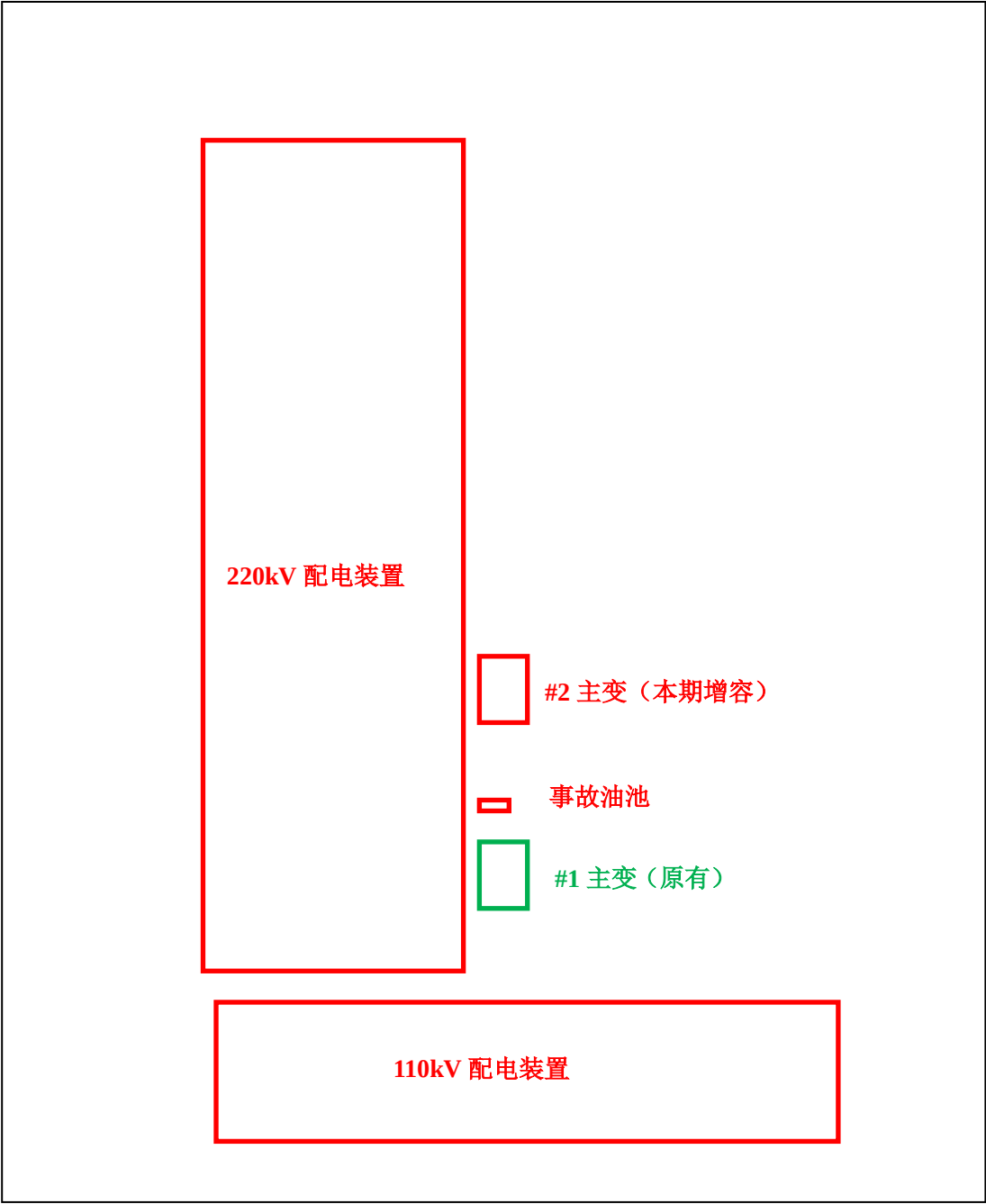
附图 3 220kV 梨园变电站总平面布置图
