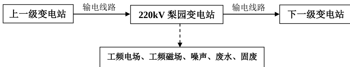
图 1 宿迁 220kV 梨园变#2 主变增容扩建工程工艺流程及产污环节示意图
