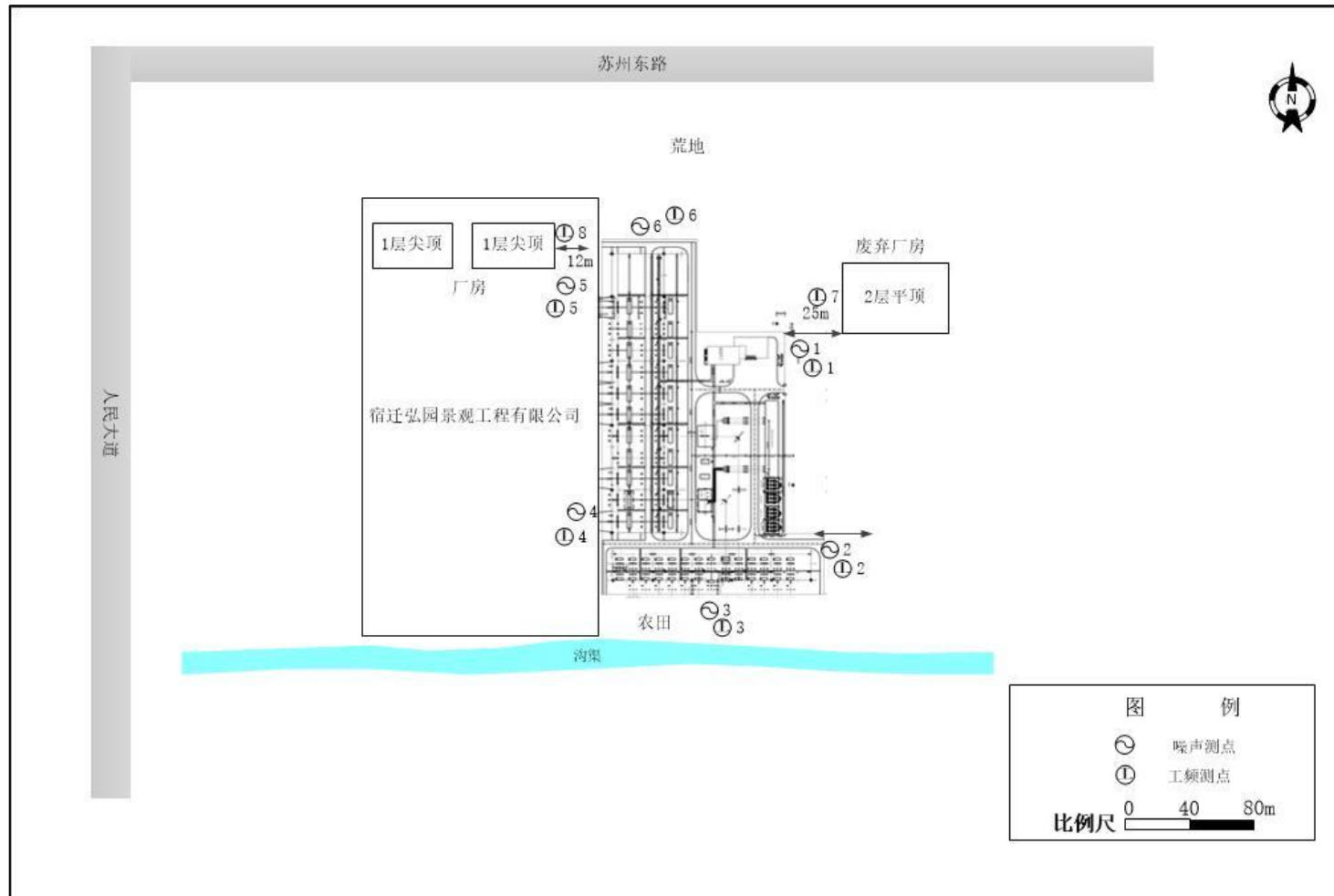
附图 2 220kV 梨园变电站监测点位及周围环境示意图
