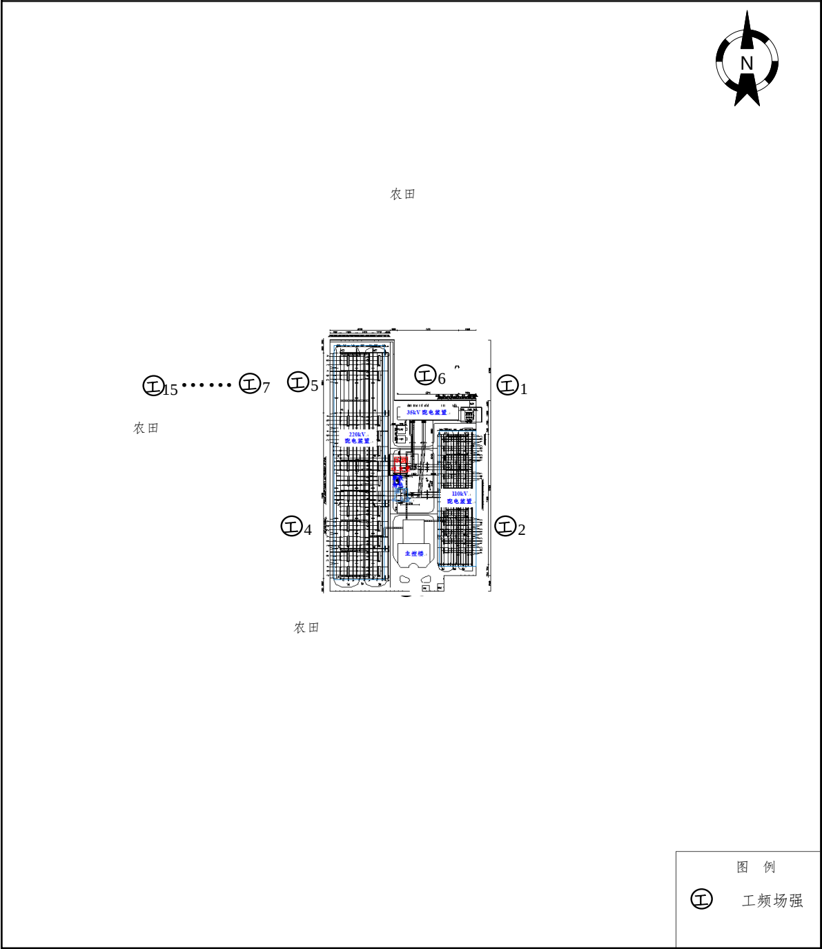
附图 4 220kV 朱桥变电站（类比站）监测点位示意图
