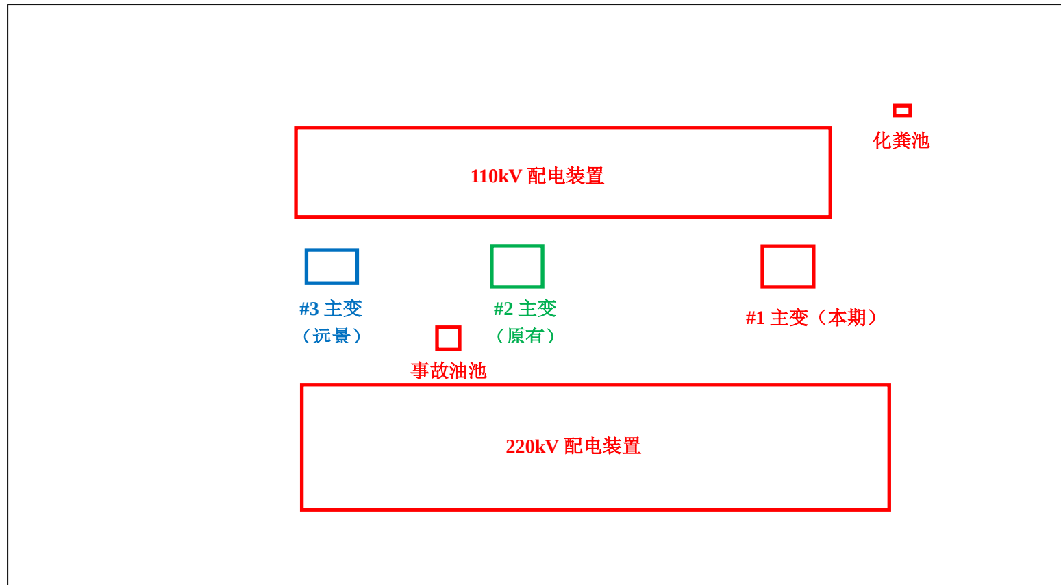
附图 3 220kV 南蔡变电站总平面布置图
