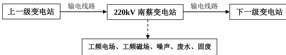
图 1 宿迁 220kV 南蔡变扩建#1 主变工程工艺流程及产污环节示意图
