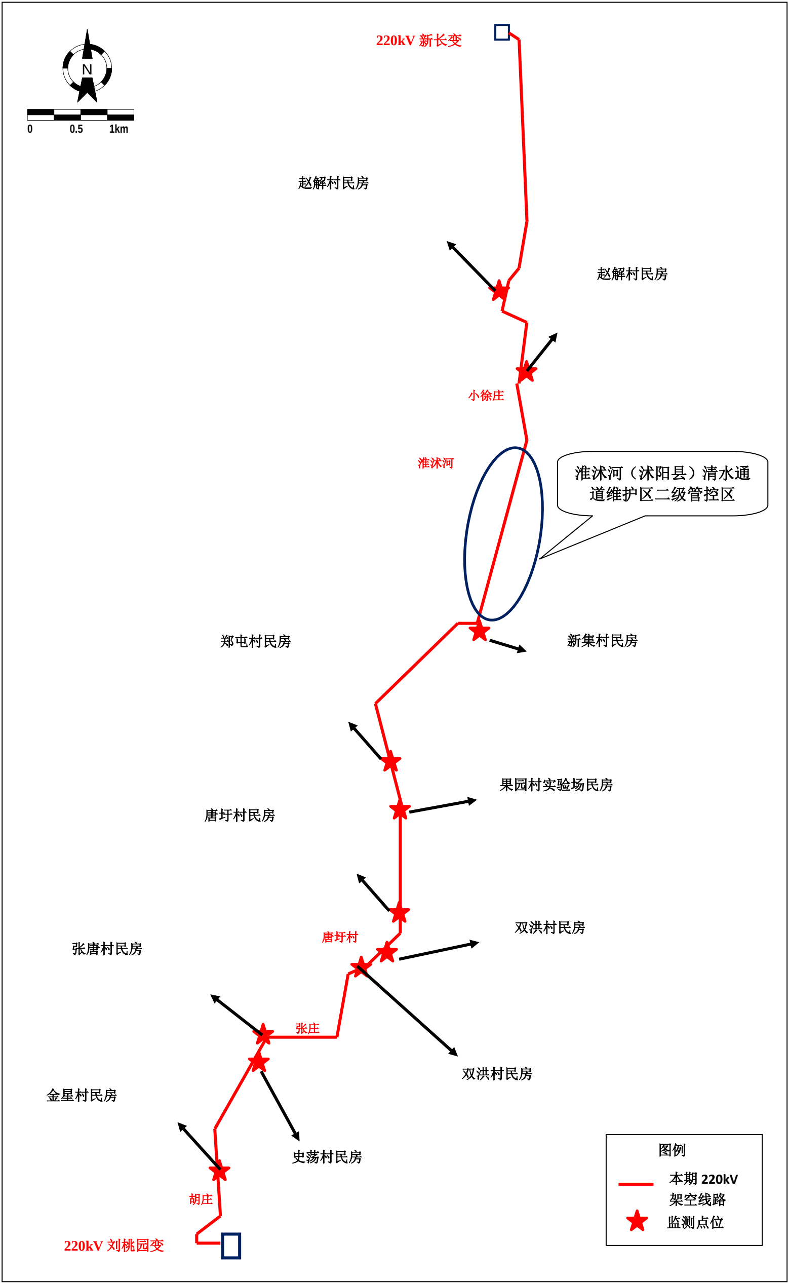
附图 2 本工程线路路径及监测点位示意图
