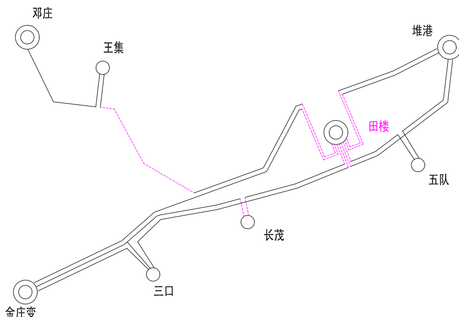
图2-1 投产年电网地理接线图
