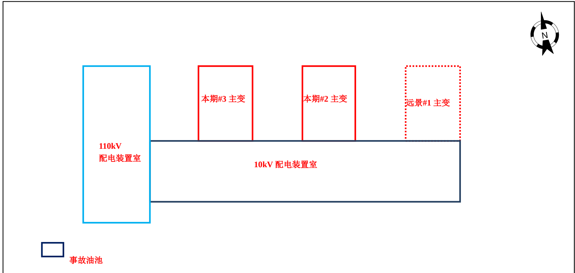
附图 3 古镇 110kV 变电站平面布置图
