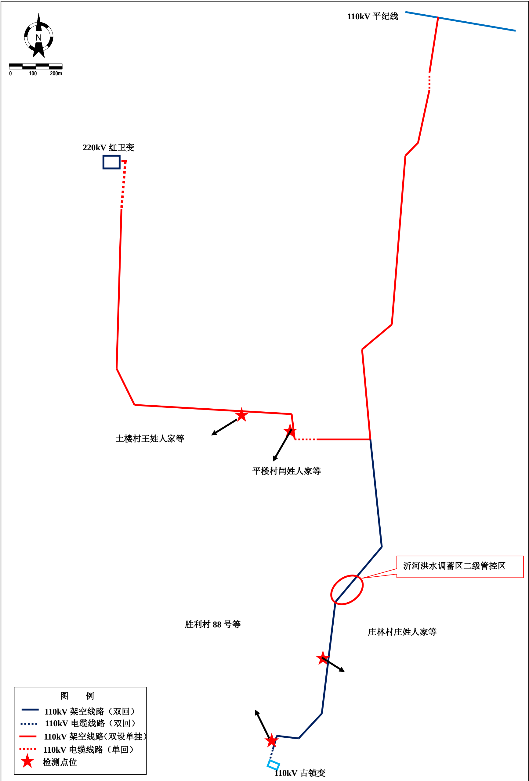
附图 4 本工程配套线路路径及检测点位示意图
