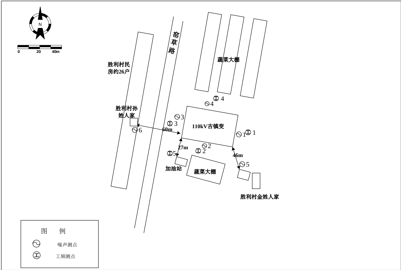
附图 2 古镇 110kV 变电站拟建址周围监测点位及环境示意图
