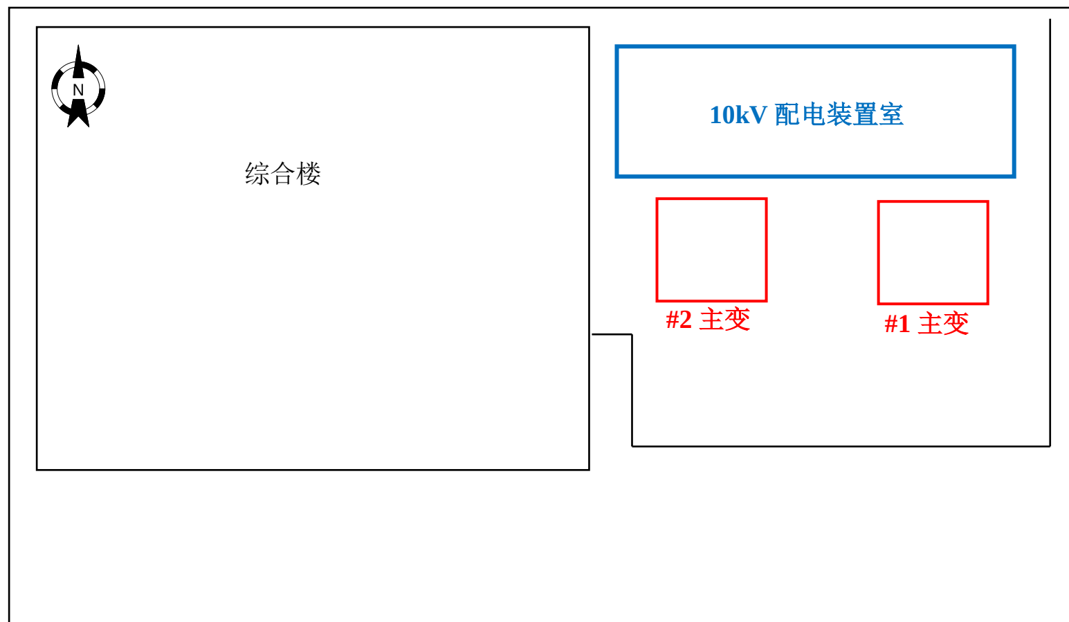
附图 3 奎山 110kV 变电站平面布置图
