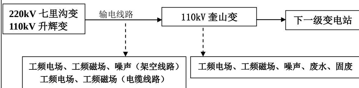
图 1 110kV 奎山变电站增容扩建工程工艺流程及产污环节示意图
