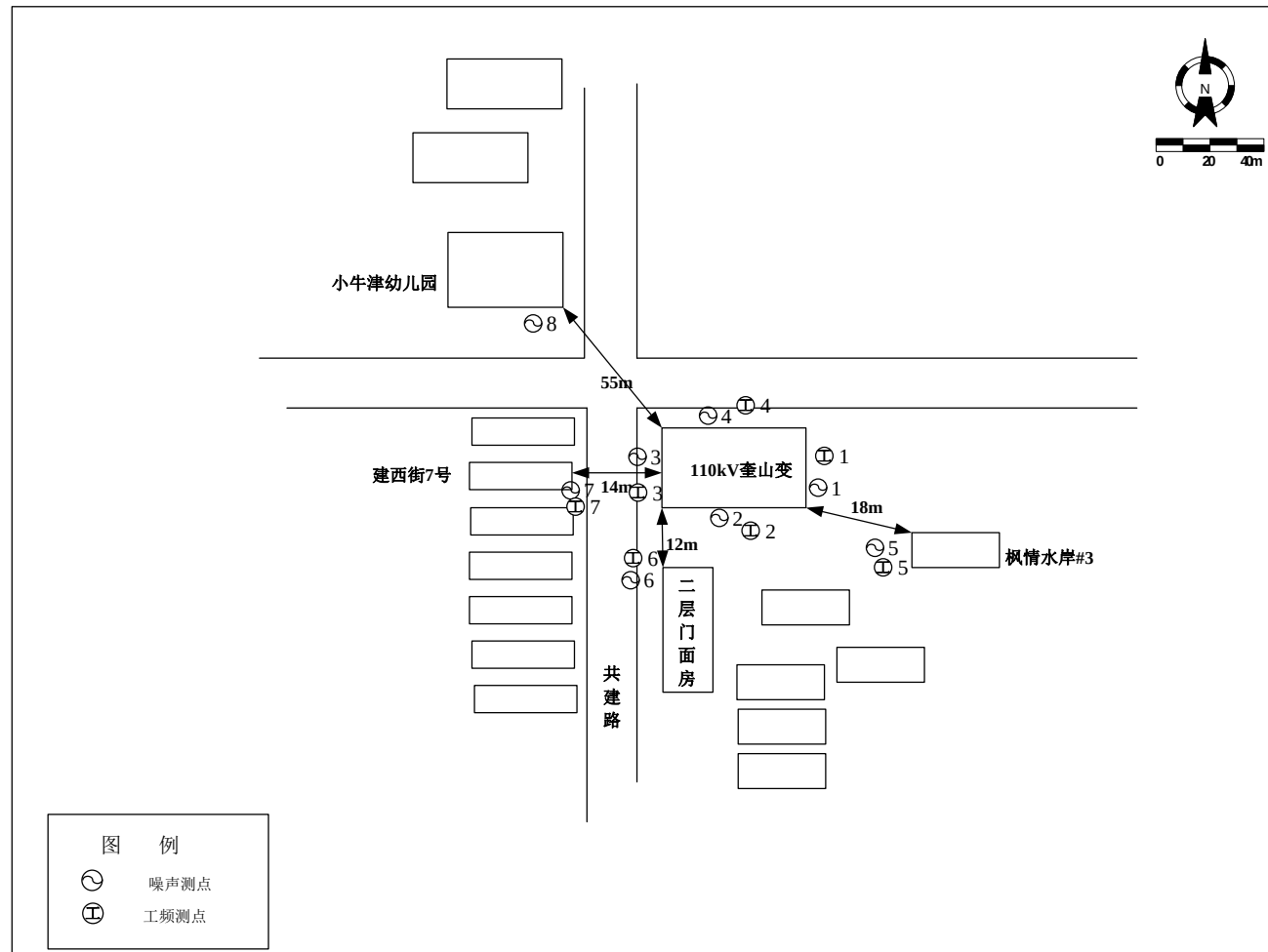
附图 2 奎山 110kV 变电站站址周围监测点位及环境示意图
