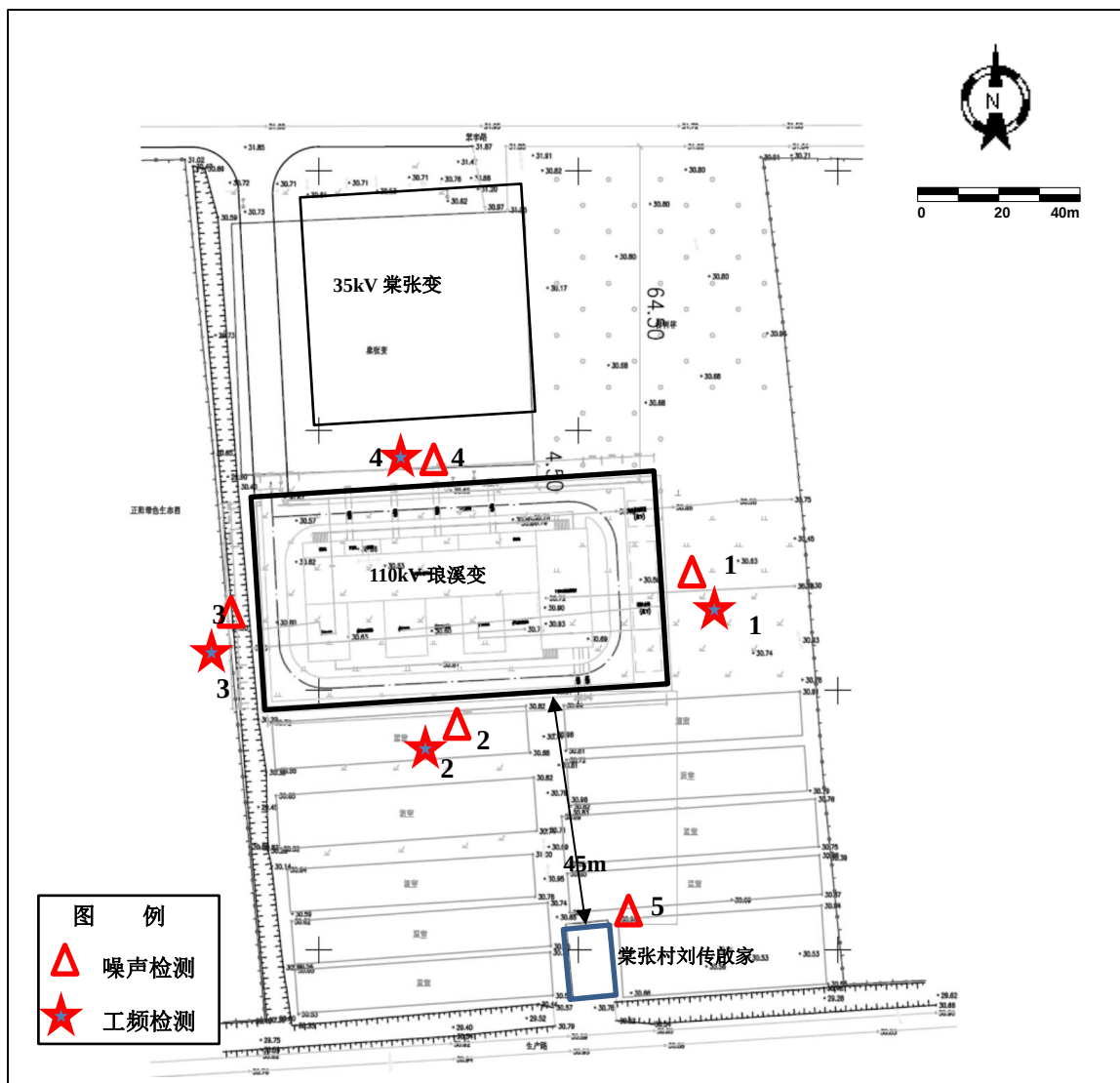
附图 2 琅溪 110kV 变电站拟建址周围监测点位及环境示意图
