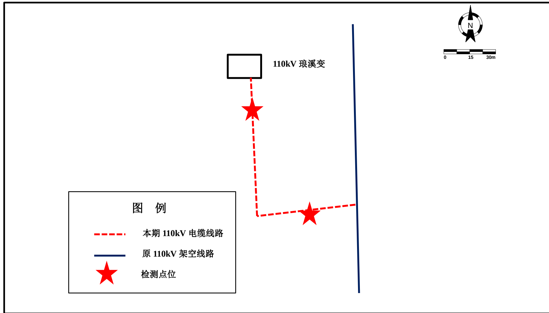
附图 4 琅溪（新区）110kV 输变电工程配套线路路径及检测点位示意图
