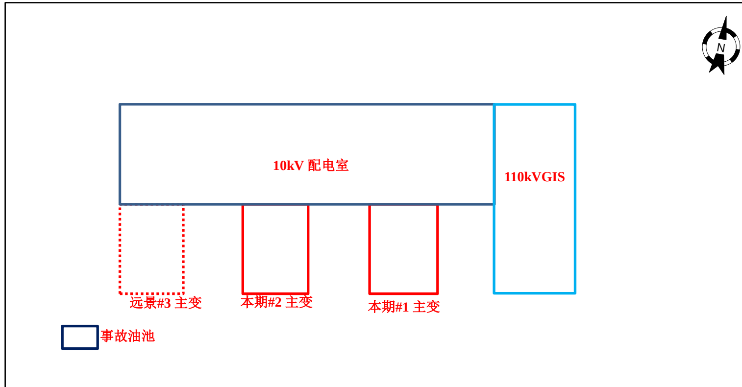
附图 3 琅溪 110kV 变电站平面布置图
