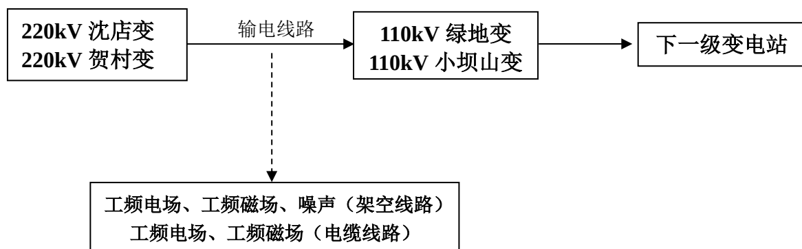
图 1 110kV 线路工程工艺流程及产污环节示意图
