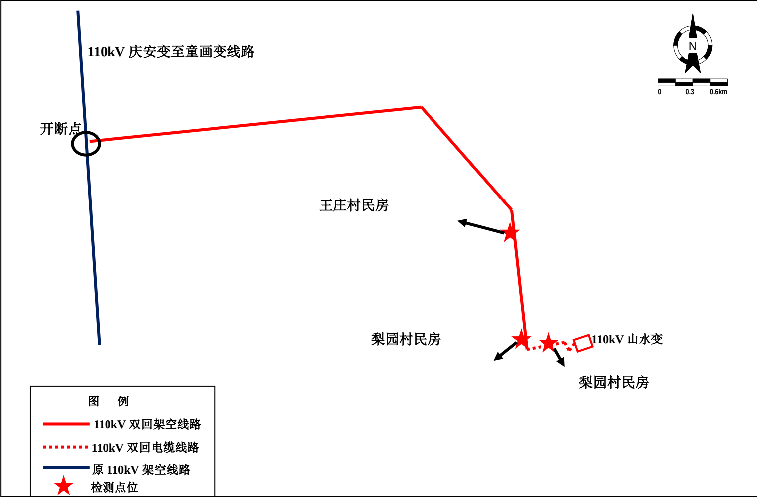
附图 4 山水（周河）110kV 输变电工程配套线路路径及检测点位示意图
