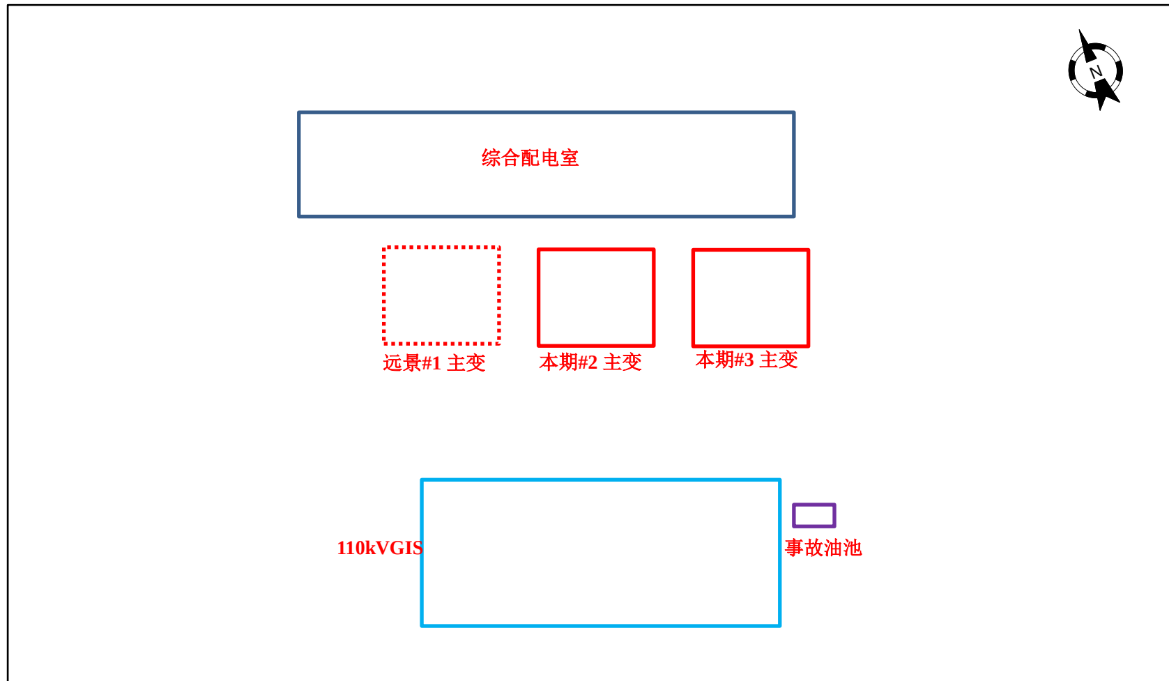
附图3 田园 110kV 变电站平面布置图
