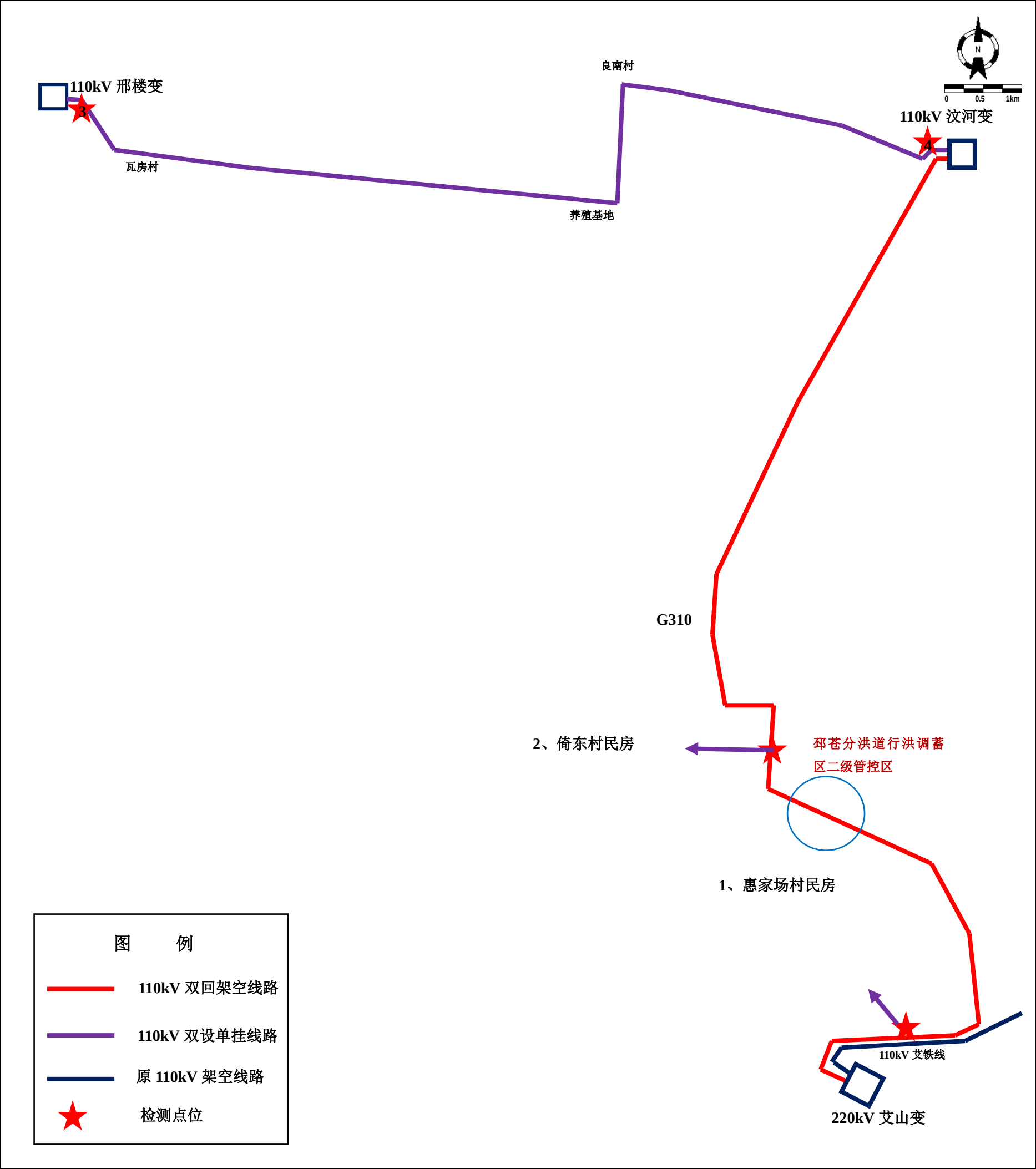
附图 4 汶河 110kV 输变电工程配套线路路径及检测点位示意图
