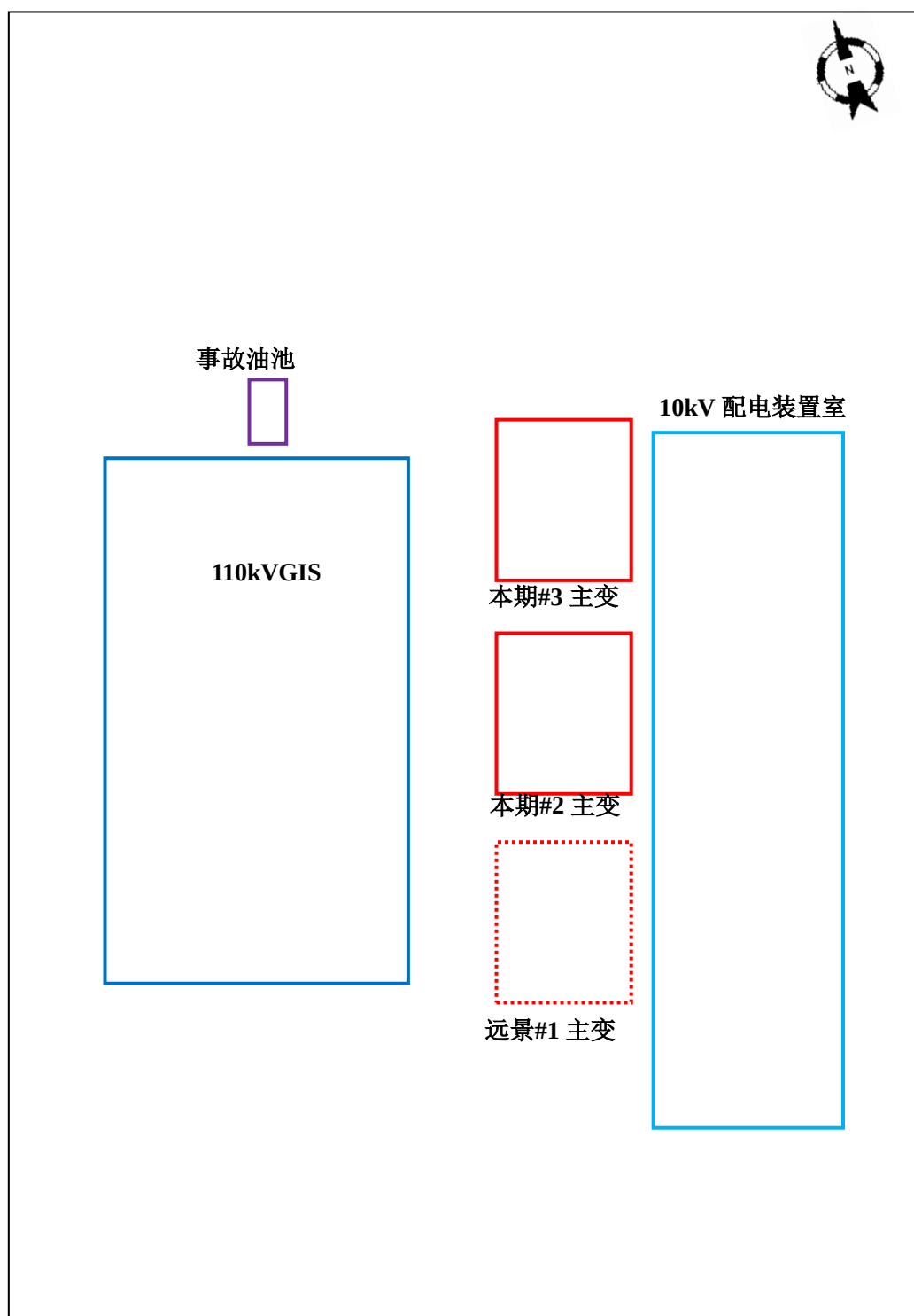
附图 3 汶河 110kV 变电站平面布置图
