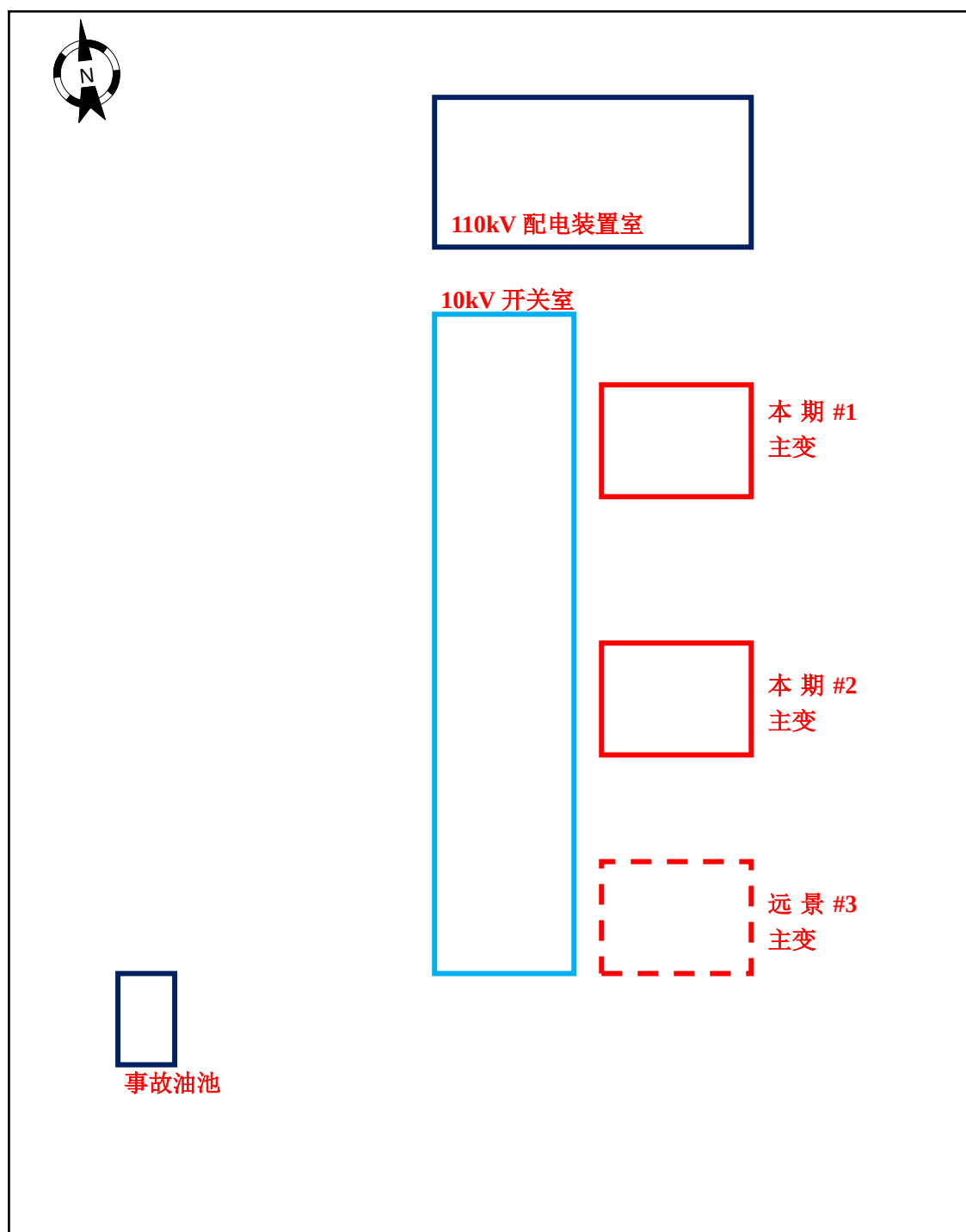
附图 3 祥和 110kV 变电站平面布置图
