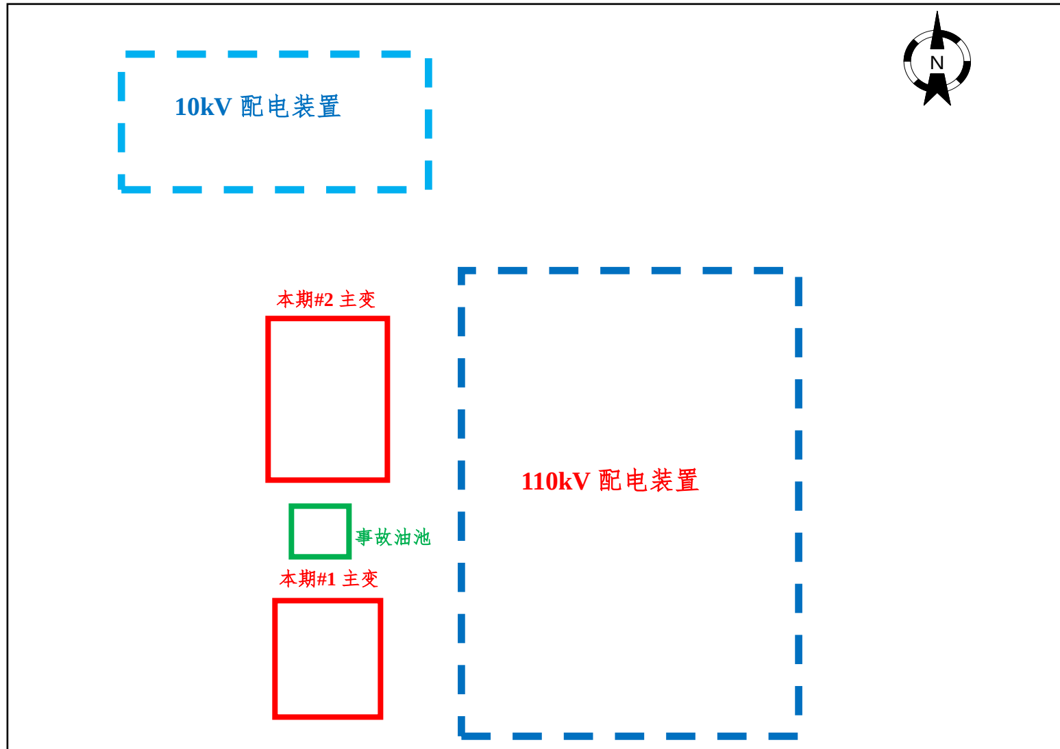
附图 3 小坝山 110kV 变电站平面布置图
