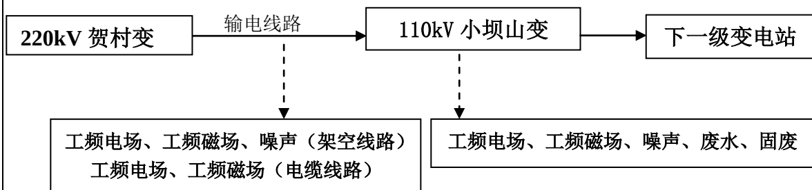
图 1 110kV 小坝山变电站增容扩建工程工艺流程及产污环节示意图 污染分析：
