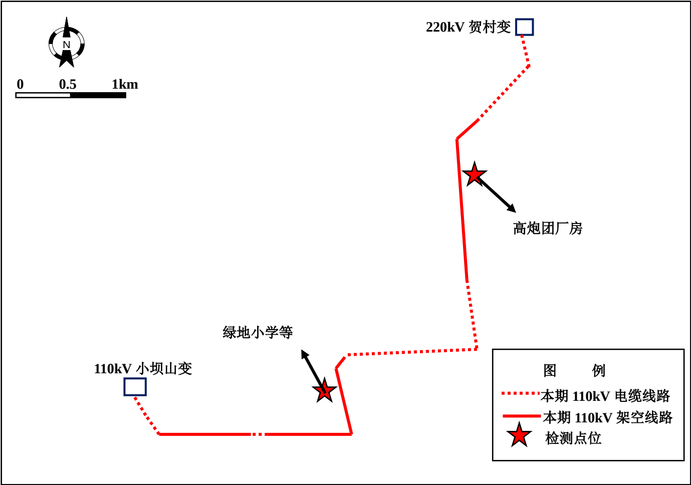
附图 4 本工程配套线路路径及检测点位示意图
