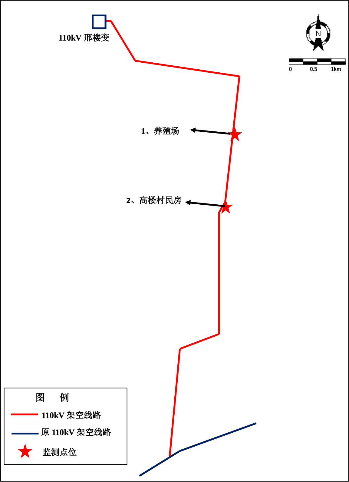
附图 4 邢楼 110kV 输变电工程配套线路路径及检测点位示意图
