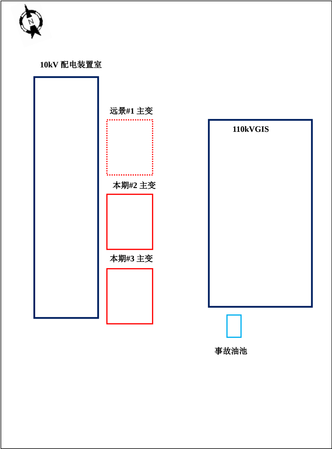
附图 3 邢楼 110kV 变电站平面布置图
