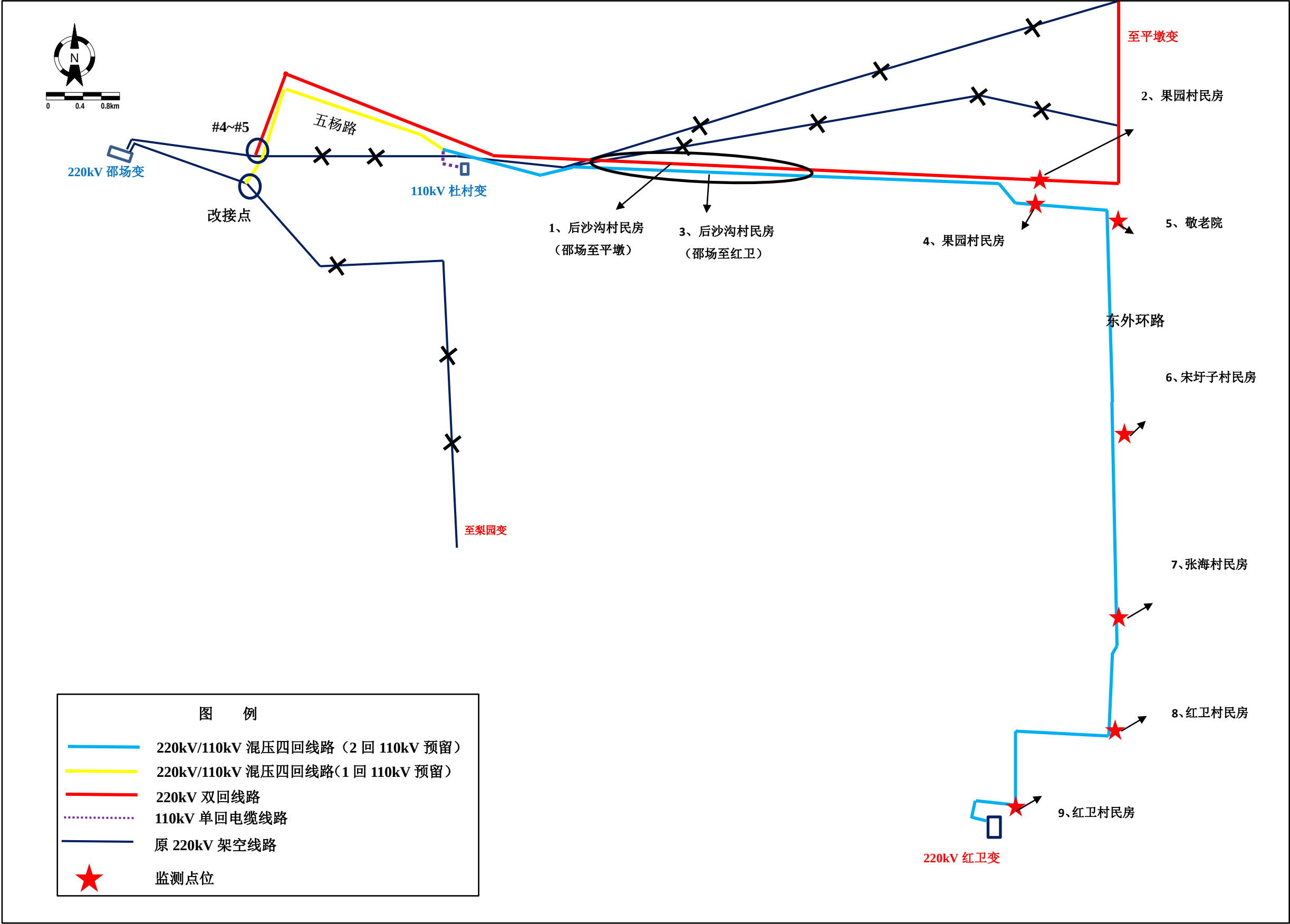
附图 2 本工程线路路径及监测点位示意图
