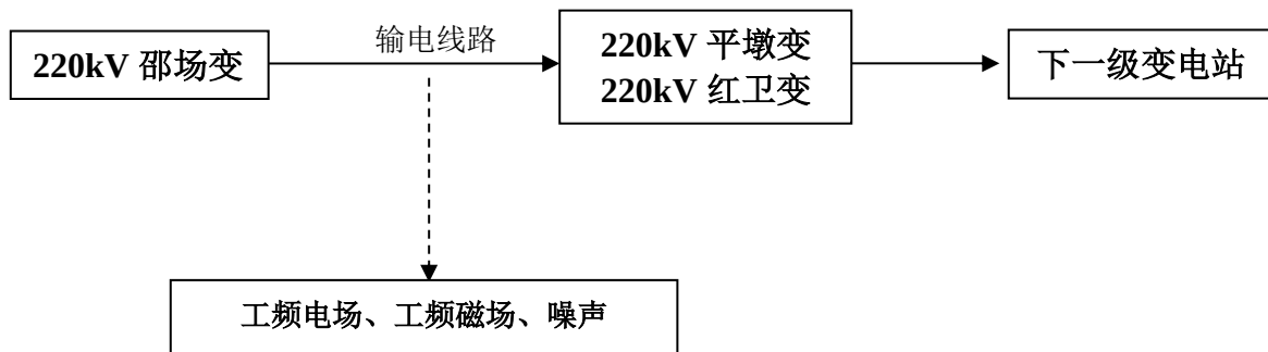
图 1 220kV 线路工程工艺流程及产污环节示意图
