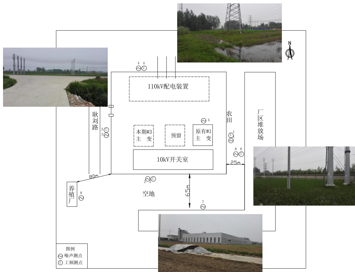
附图 2 110kV 黄竹变电站监测点位及周围环境示意图
