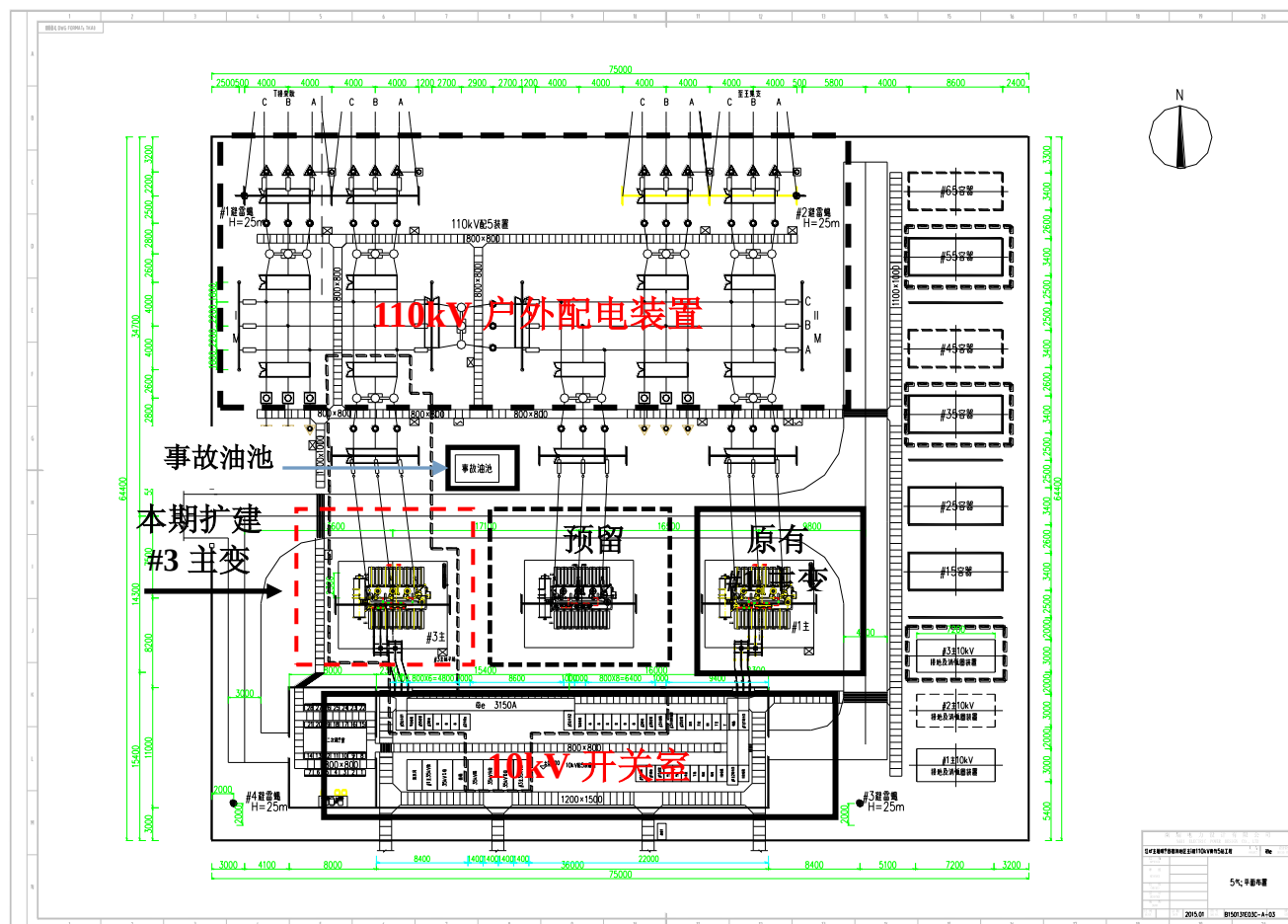
图 3 110kV 黄竹变电站平面布置示意图
