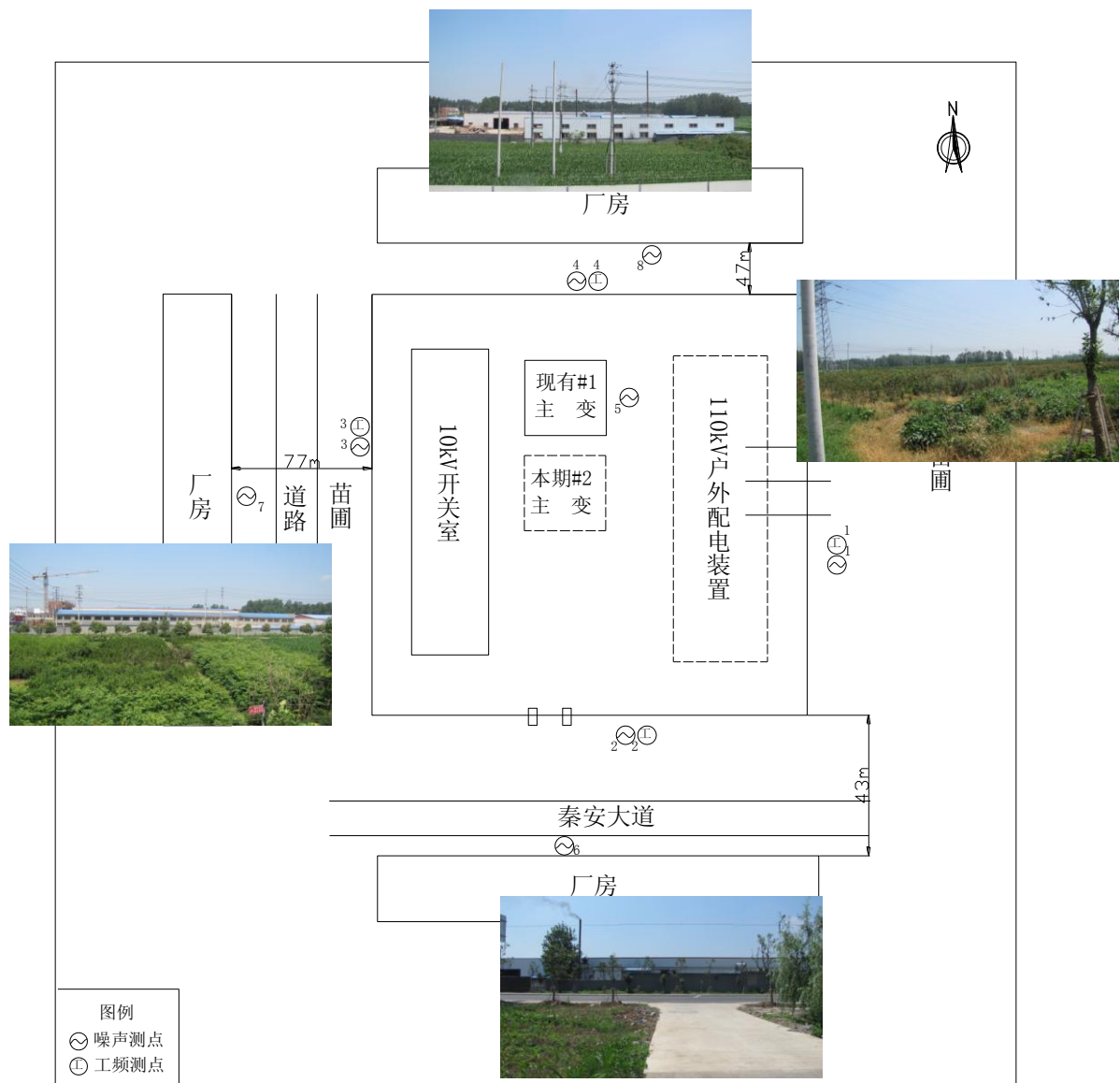
附图 2 110kV 贤官变电站监测点位及周围环境示意图
