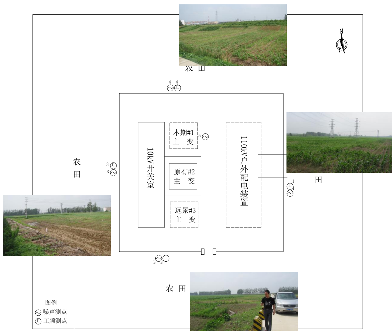
附图 2 110kV 梅花变电站监测点位及周围环境示意图
