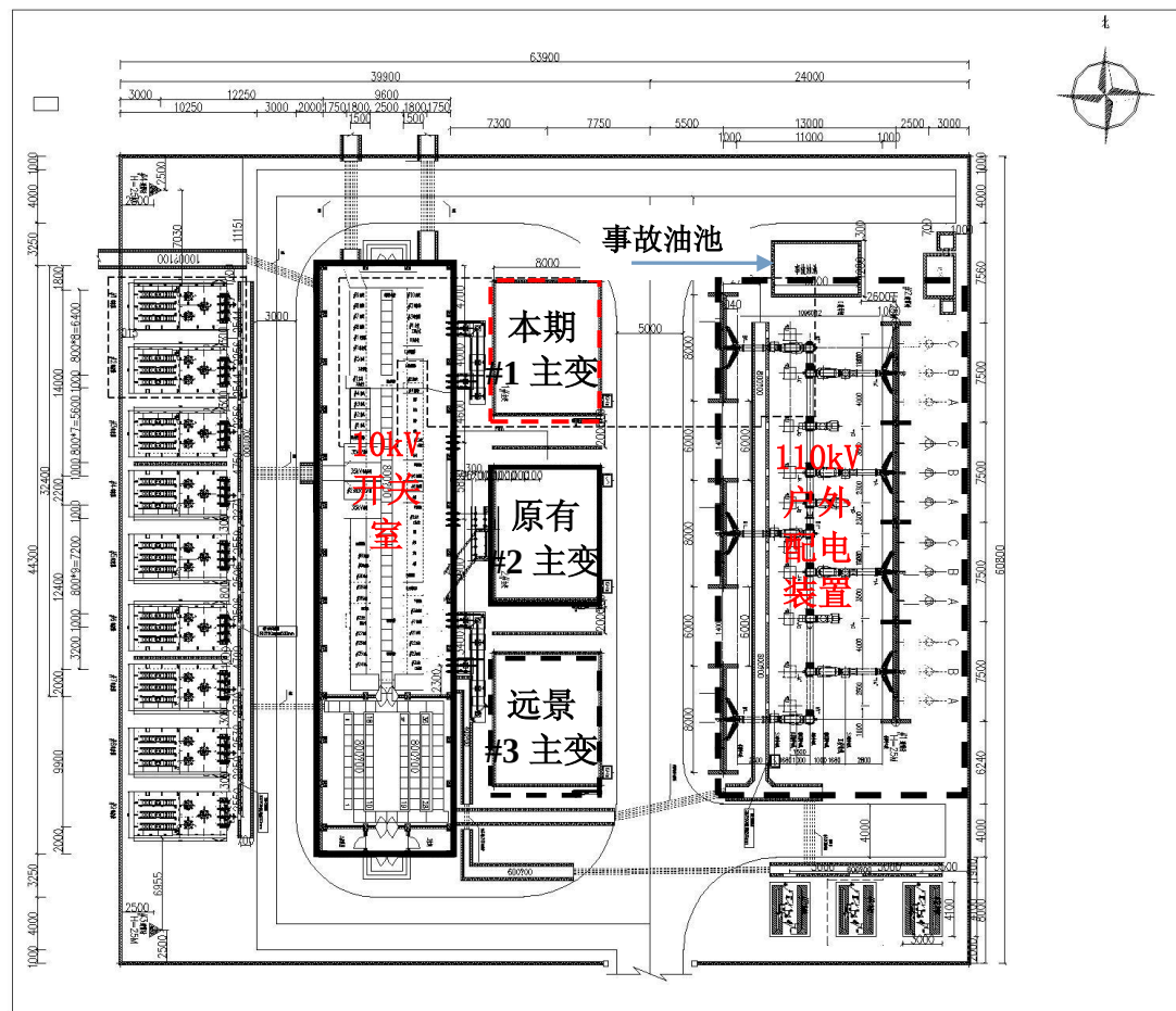
附图 3 110kV 梅花变电站平面布置示意图
