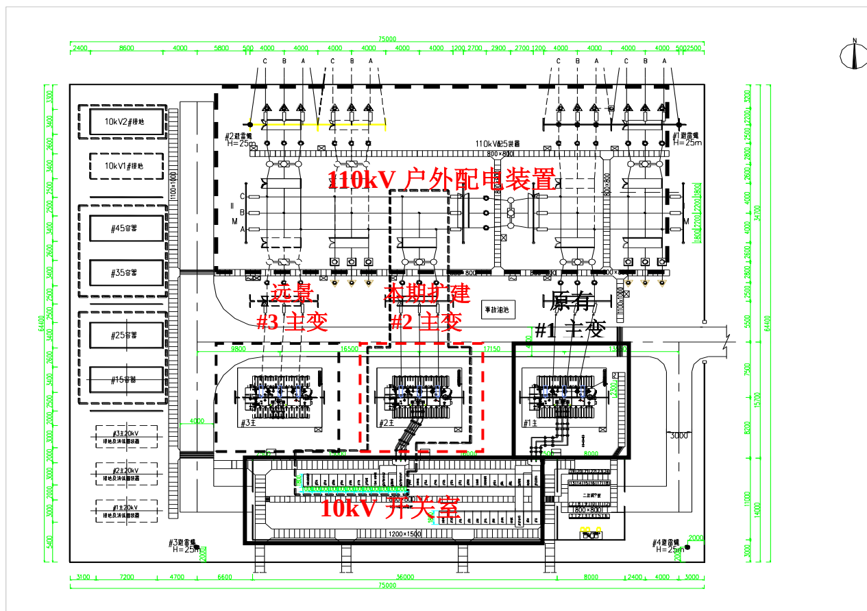
附图 3 110kV 北庄变电站平面布置示意图
