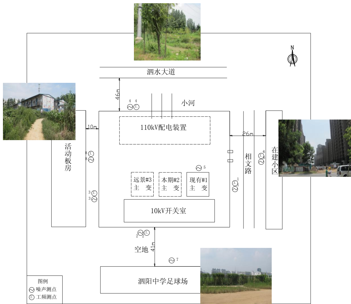
附图 2 110kV 北庄变电站监测点位及周围环境示意图
