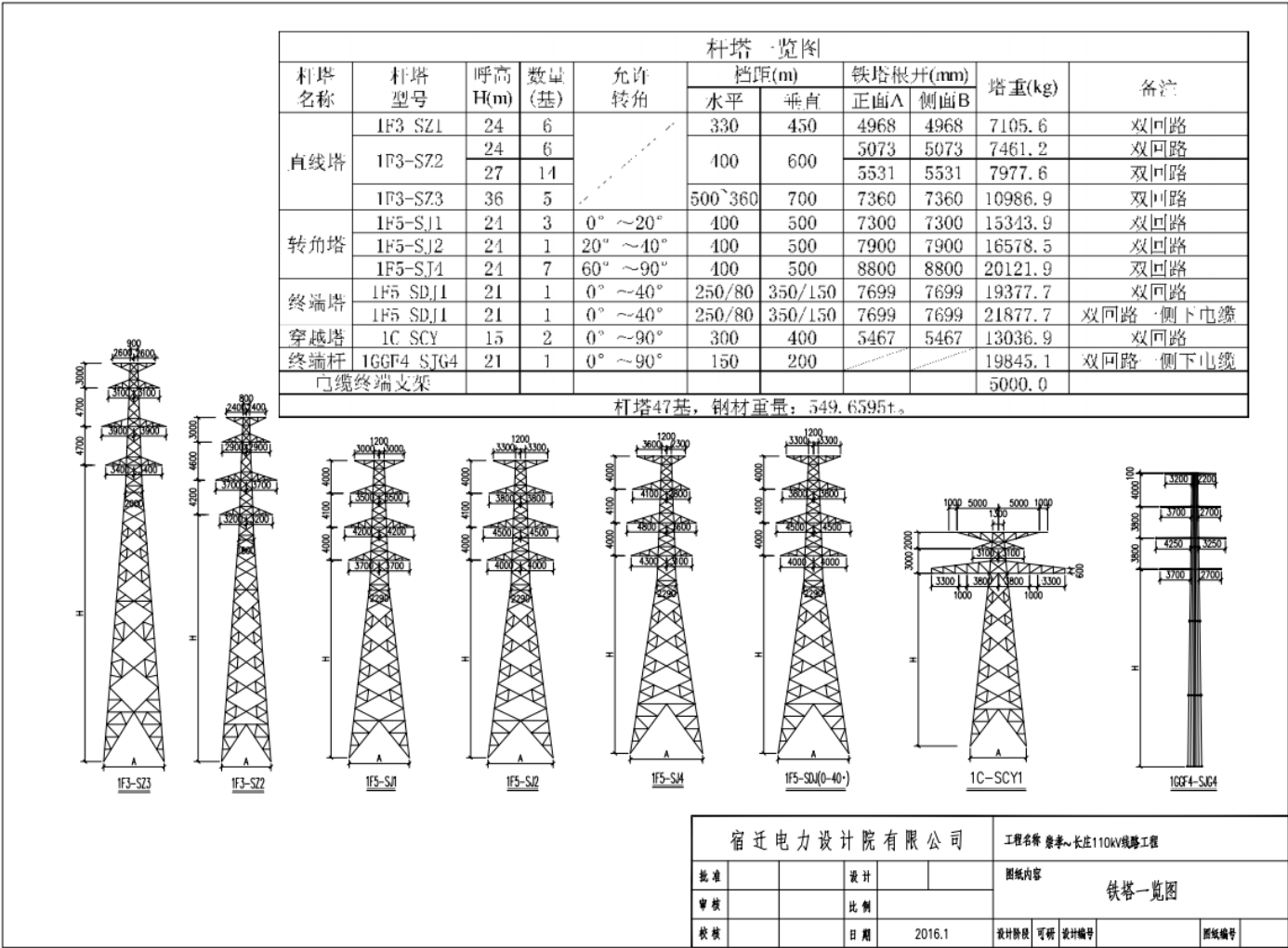
附图 4-3 崇孝变至长庄变 110kV 线路工程塔型图
