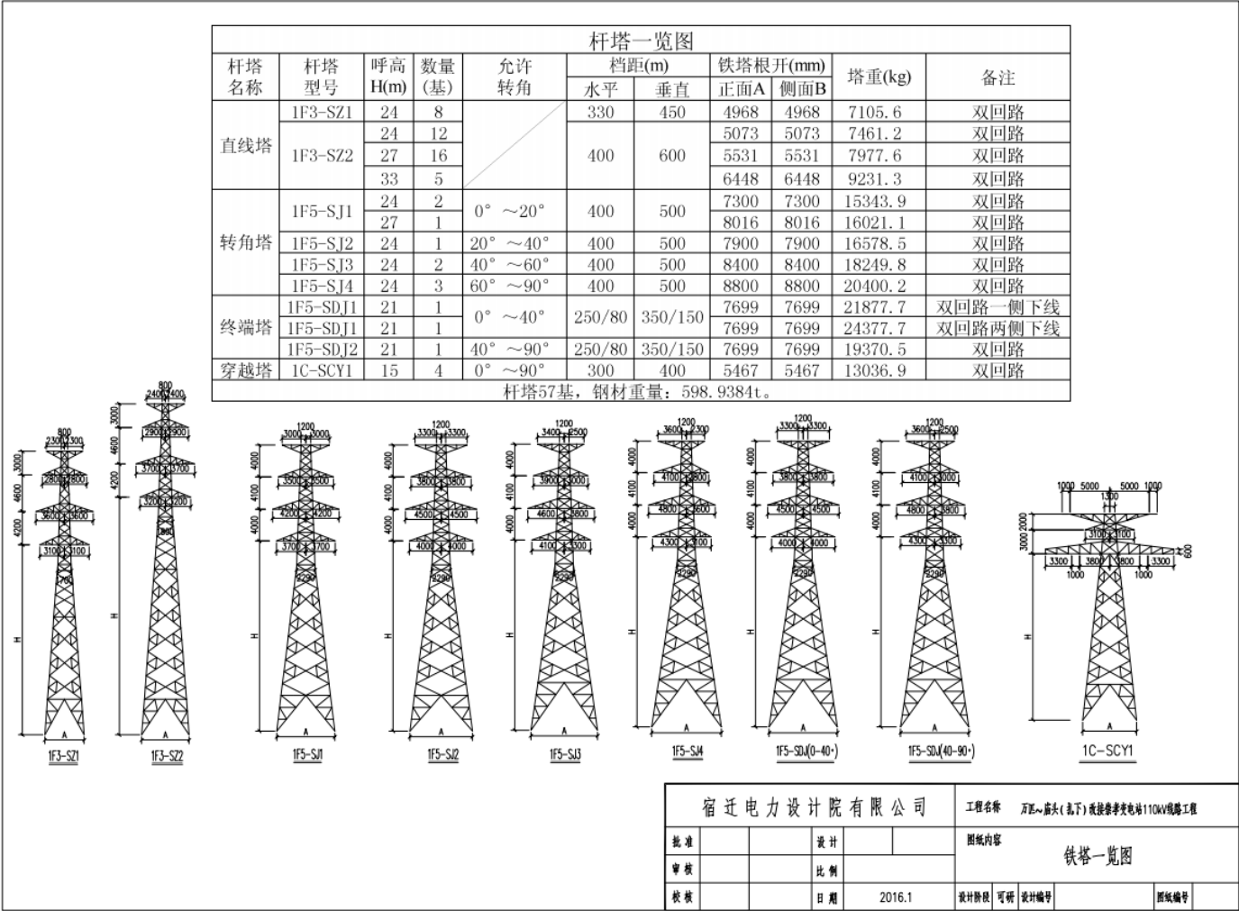
附图 4-1 万匹变至庙头（扎下）变、万匹变至贤官变改接崇孝变电站 110kV 线路工程塔型图
