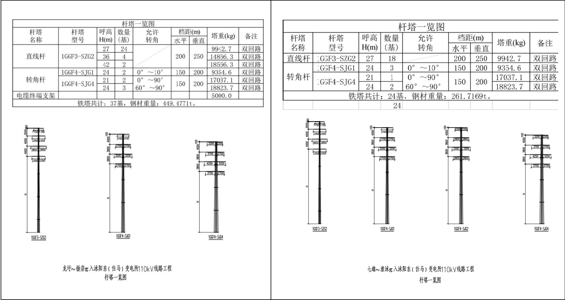
附图 3 本工程塔型图
