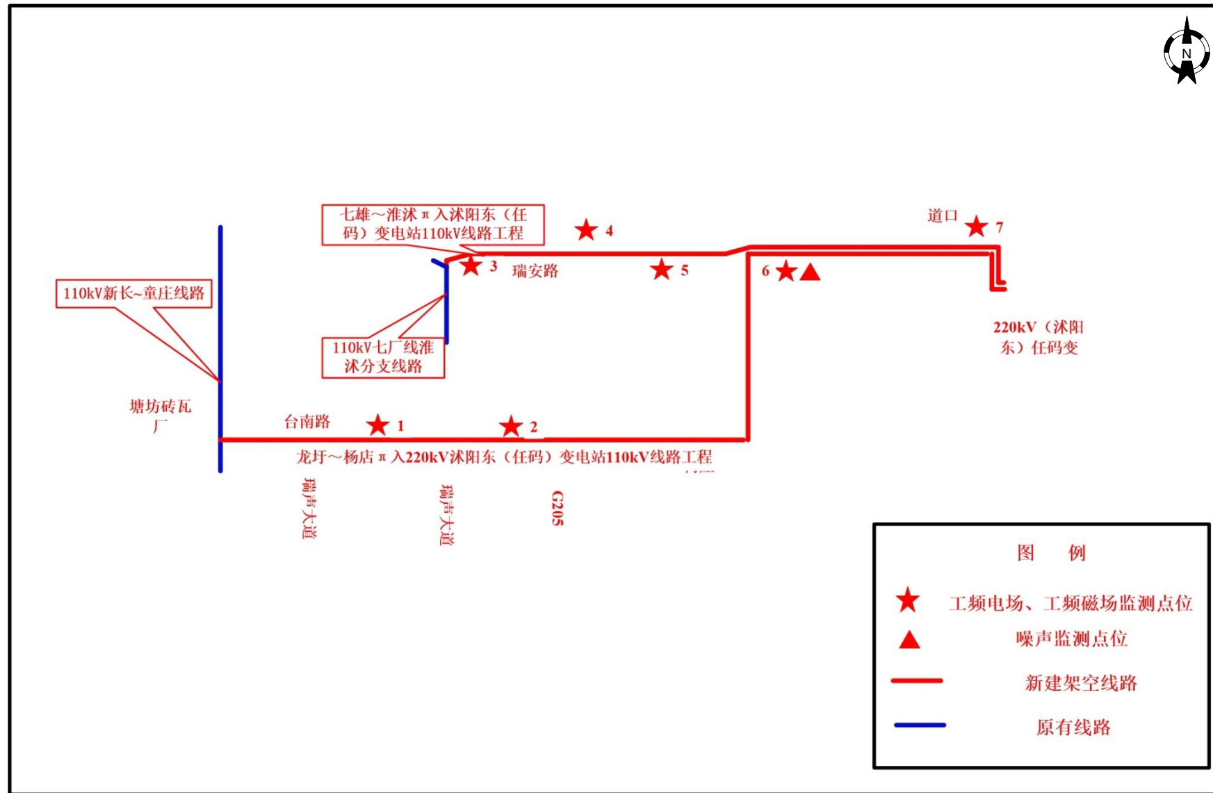
附图 2 沭阳 220kV 沭阳东（任码）变电站 110kV 送出工程线路路径及监测点位示意图
