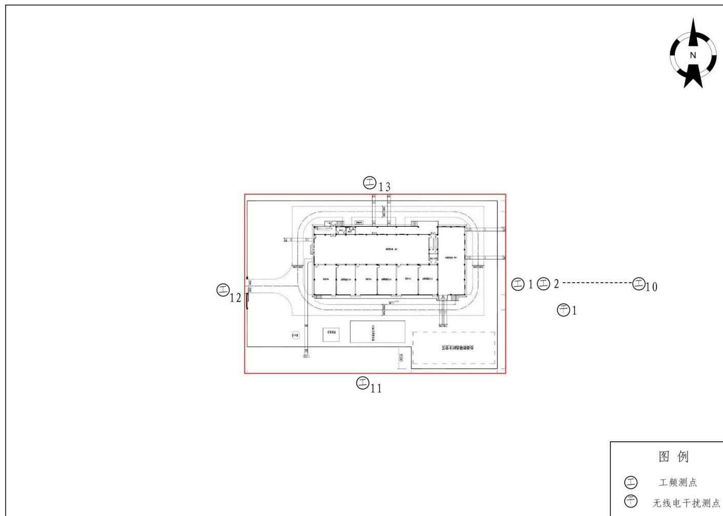
附图 5 110kV 青桥变电站（类比站）监测点位示意图
