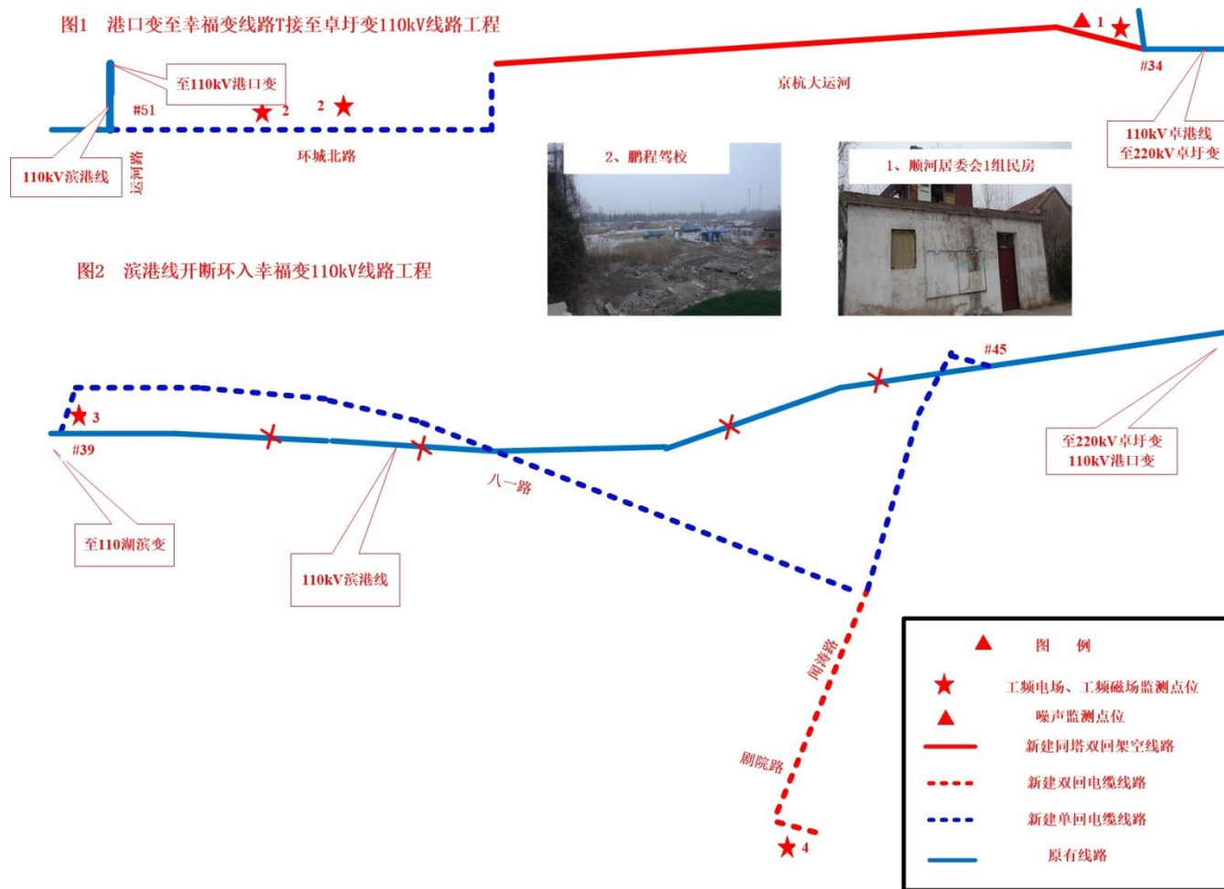
附图 4 110kV 幸福变电站配套 110kV 线路路径及监测点位示意图
