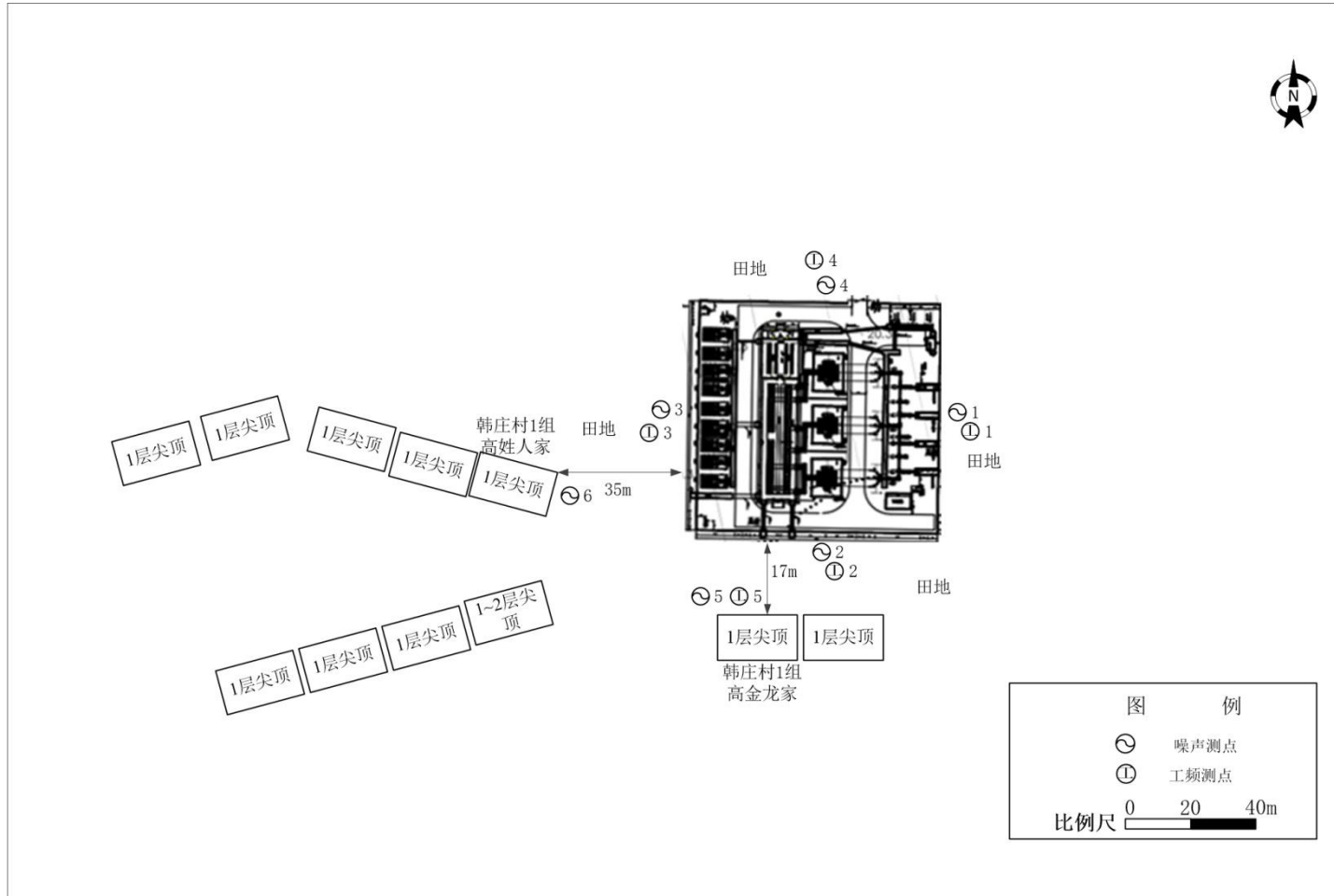
附图 2 110kV 振兴变电站拟建址周围监测点位及环境示意图
