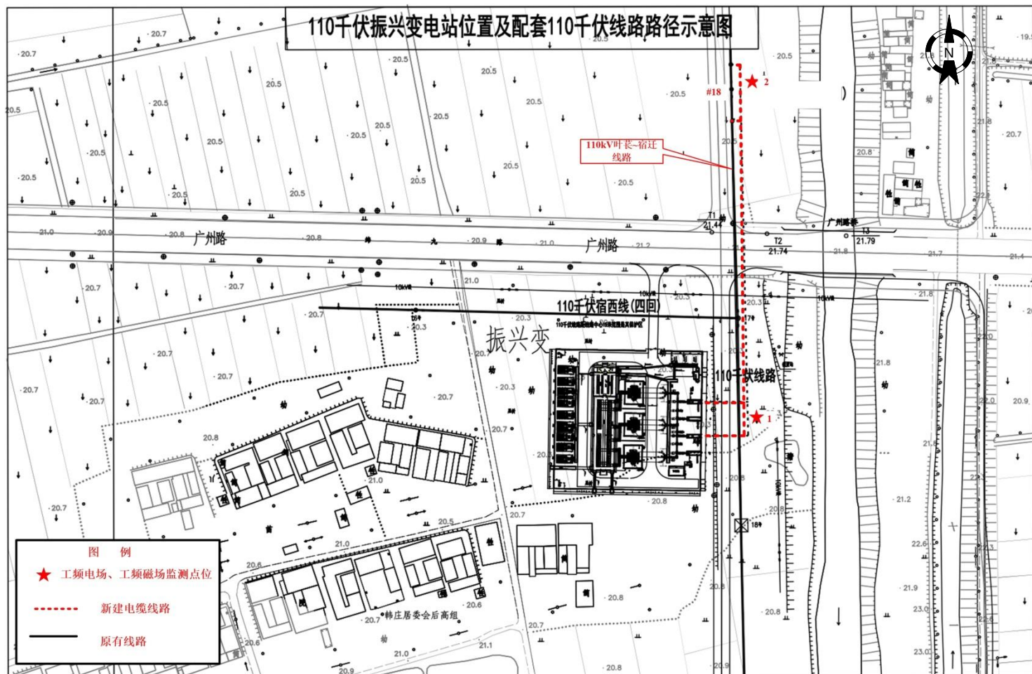
附图 4 110kV 振兴变电站配套 110kV 线路路径及监测点位示意图
