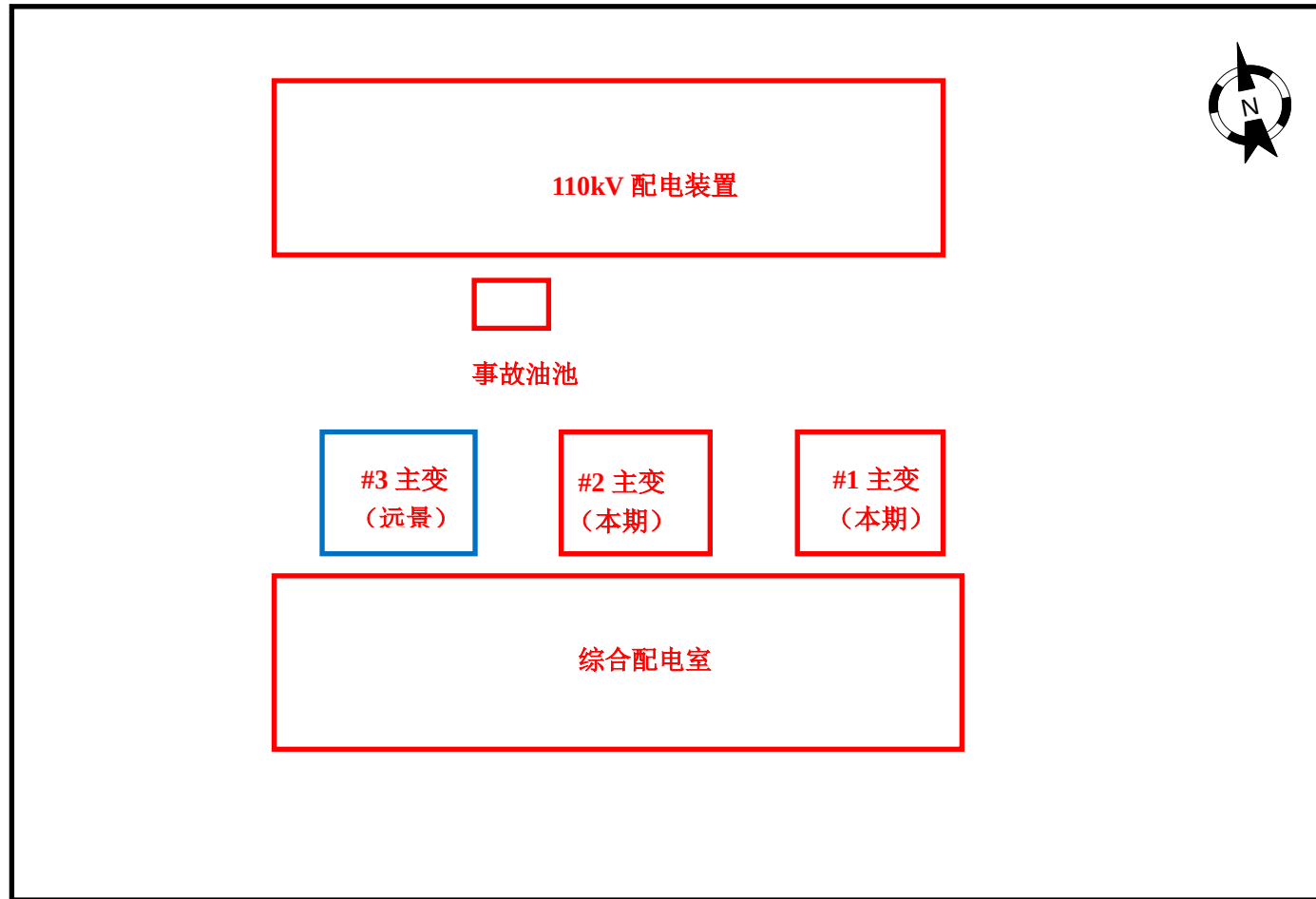
附图 3 110kV 北区变电站总平面布置图
