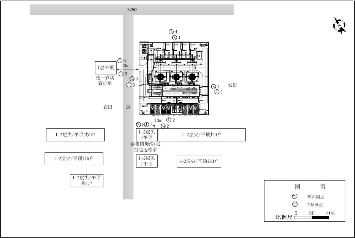
附图 2 110kV 蔡集变电站监测点位及周围环境示意图
