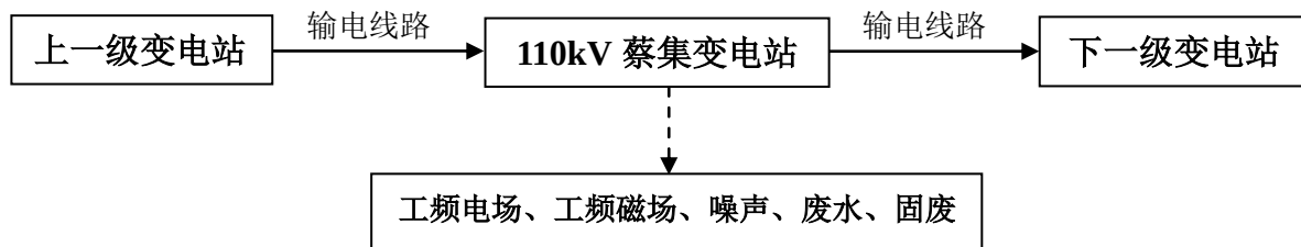
图 1 宿迁 110kV 蔡集变电站扩建#1 主变工程工艺流程及产污环节示意图
