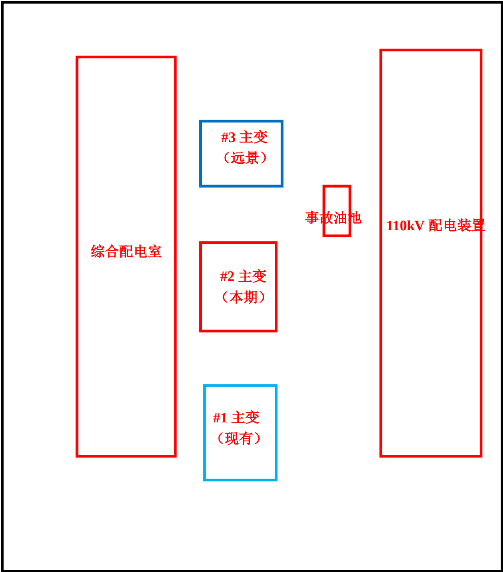
附图 3 110kV 果园变电站总平面布置图
