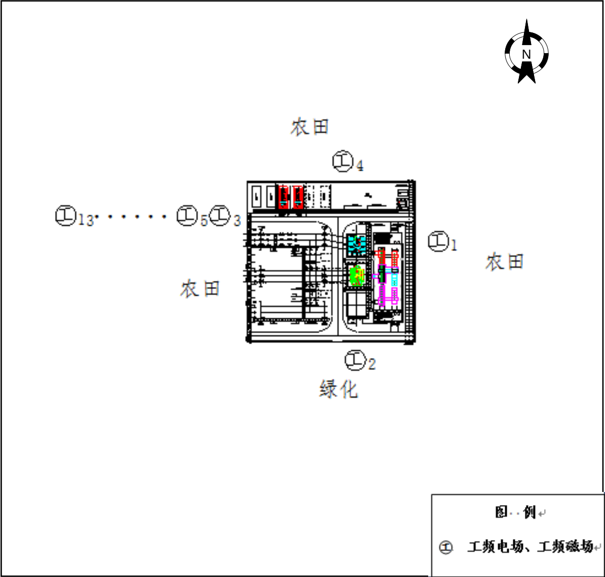
附图 4 110kV 练湖变电站（类比站）监测点位示意图
