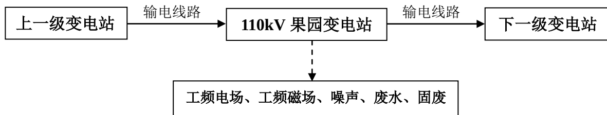
图 1 宿迁 110kV 果园变电站扩建#2 主变工程工艺流程及产污环节示意图
