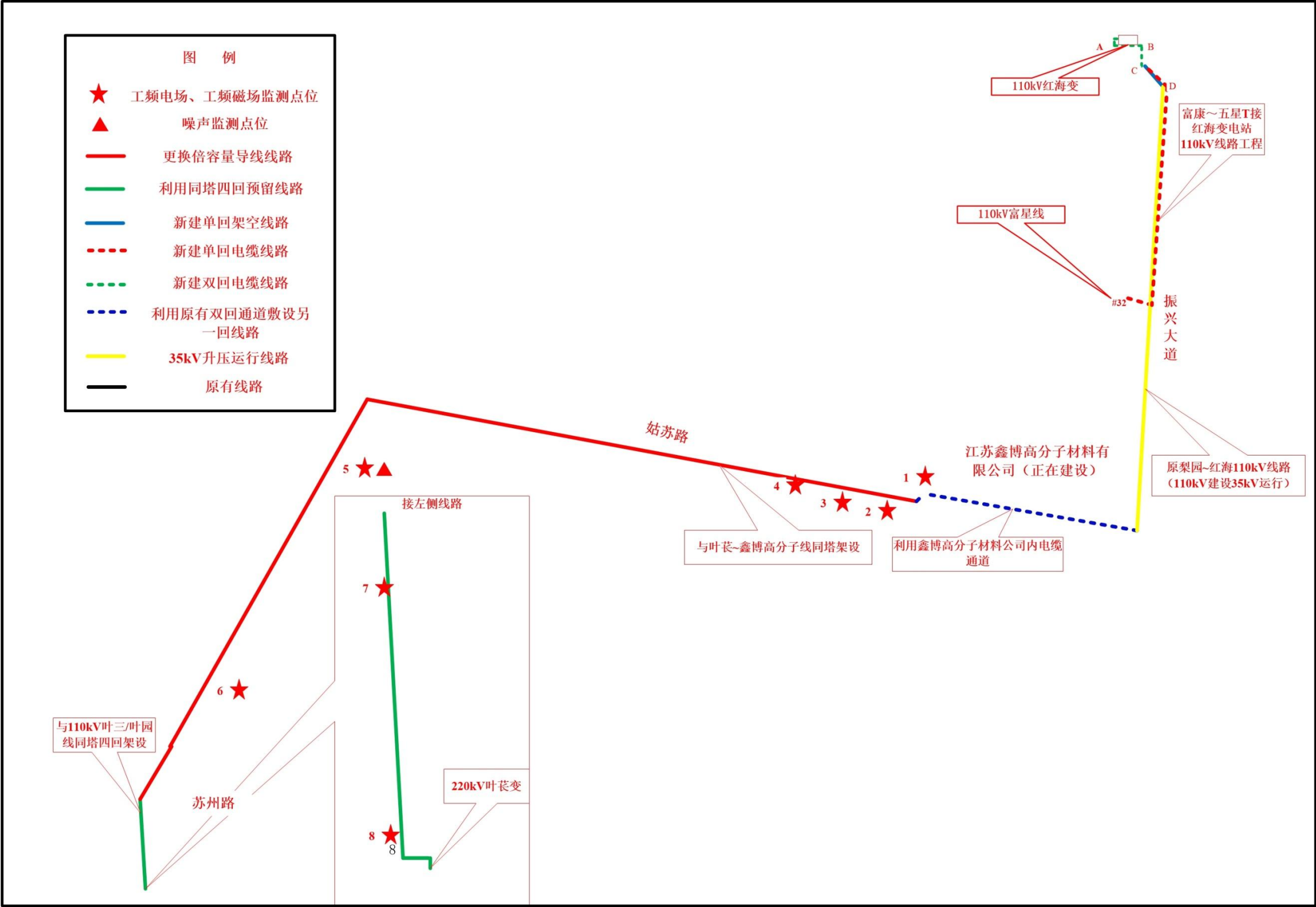
附图 4 110kV 红海变电站配套 110kV 线路路径及监测点位示意图
