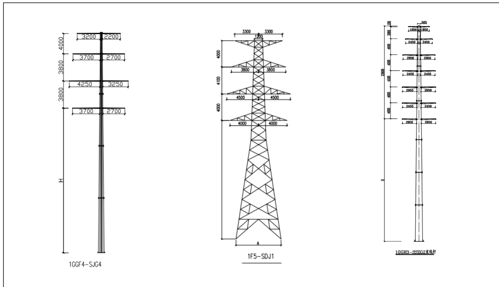
附图 5 本工程塔型图
