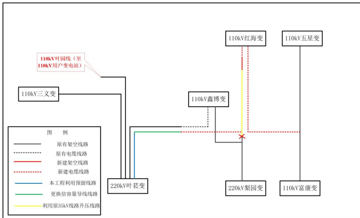
图 1 本工程接线示意图
