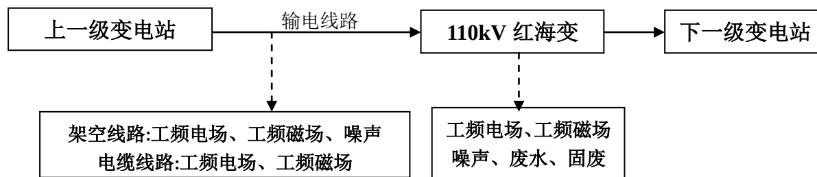
图 2 110kV 输变电工程工艺流程及产污环节示意图
