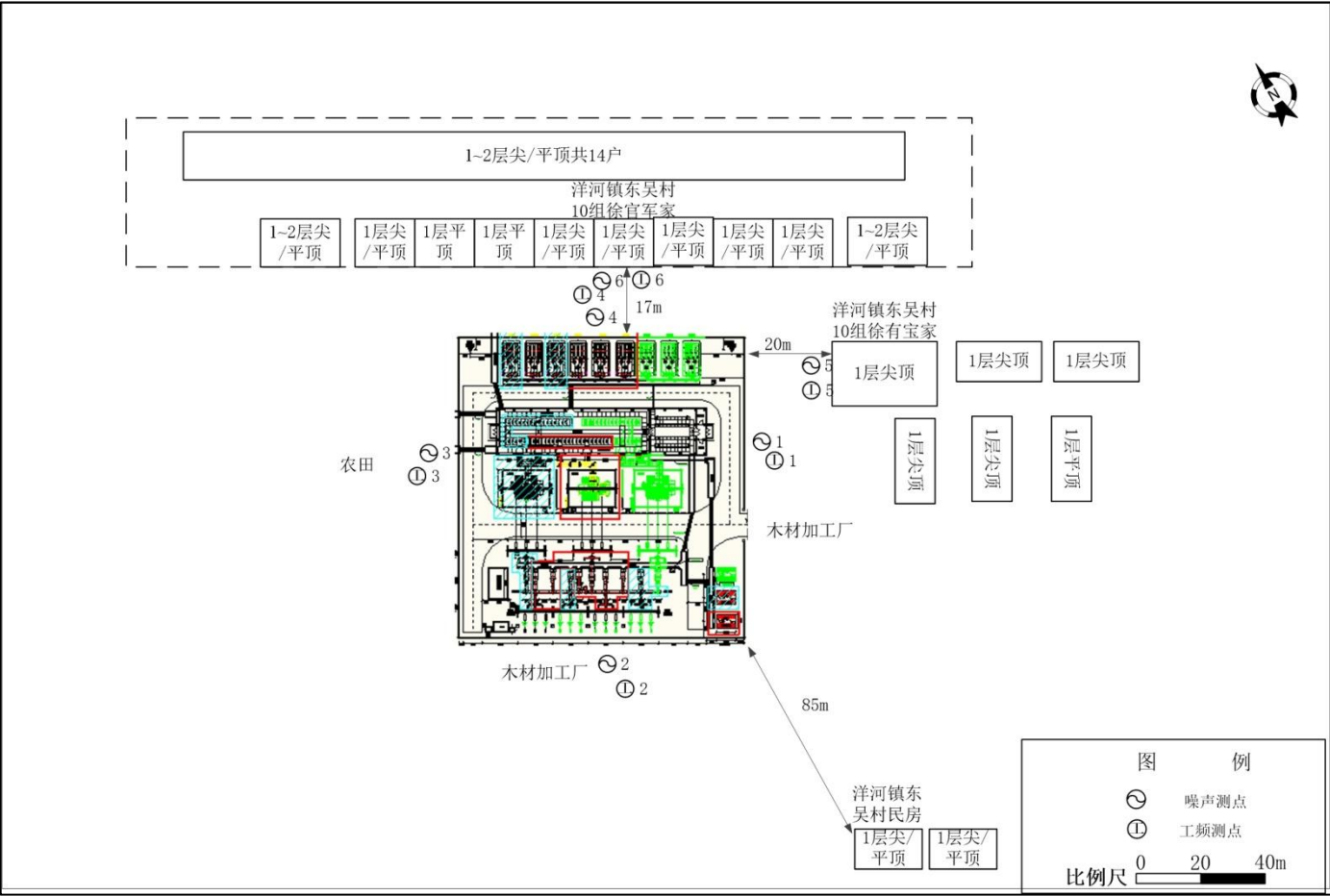
附图 2 110kV 新城变电站监测点位及周围环境示意图
