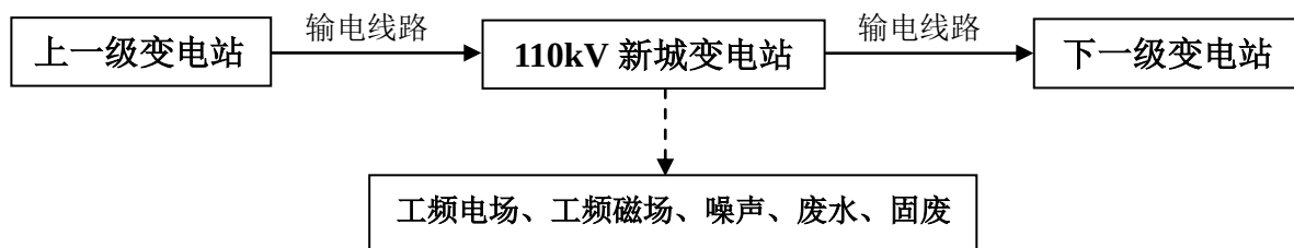
图 1 宿迁 110kV 新城变电站扩建#1 主变工程工艺流程及产污环节示意图
