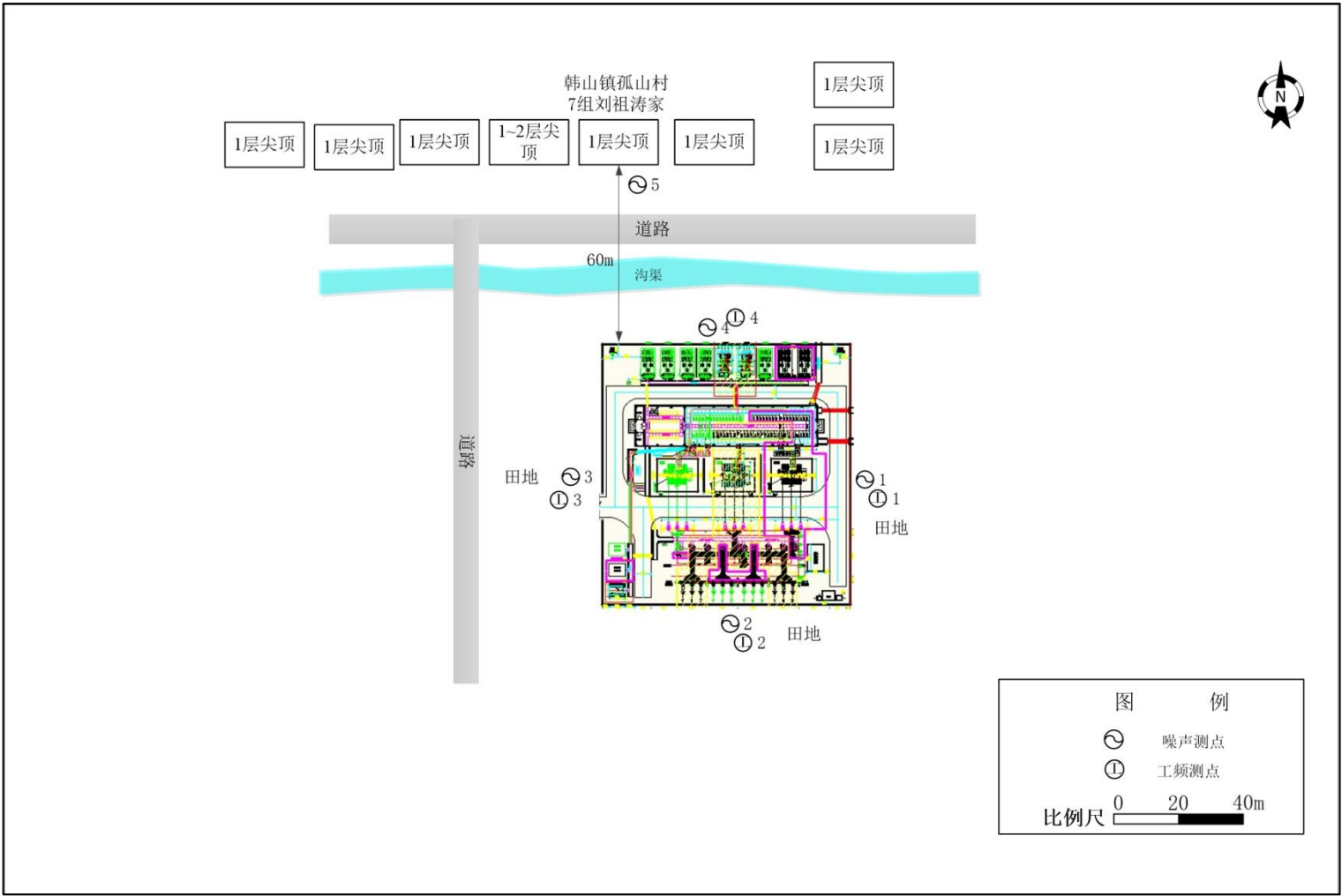
附图 2 110kV 韩山变电站监测点位及周围环境示意图
