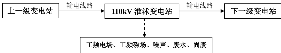
图 1 沭阳 110kV 淮沭变电站扩建#2 主变工程工艺流程及产污环节示意图
