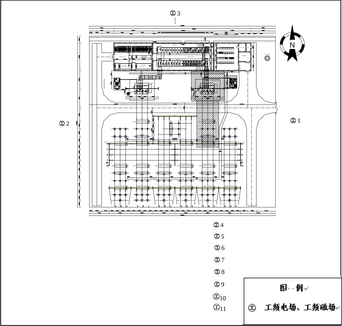
附图 4 110kV 邓码变电站（类比站）监测点位示意图
