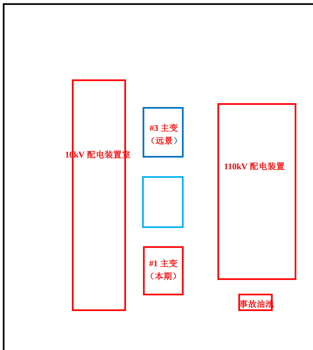
附图 3 110kV 茆圩变电站总平面布置图
