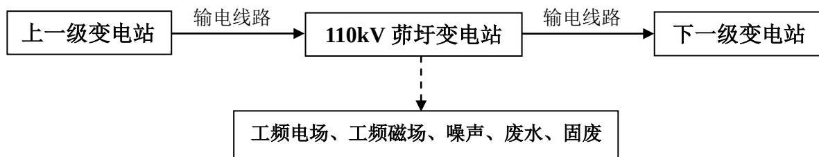
图 1 沭阳 110kV 茆圩变电站扩建#1 主变工程工艺流程及产污环节示意图
