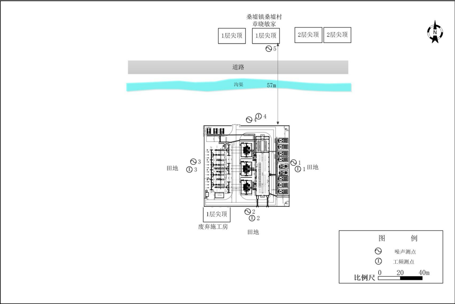
附图 2 110kV 桑墟变电站监测点位及周围环境示意图
