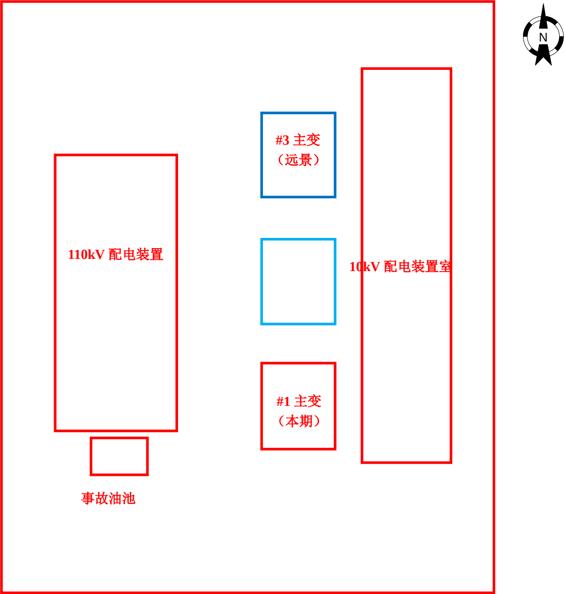
附图 3 110kV 桑墟变电站总平面布置图
