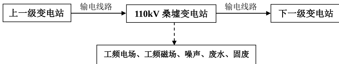
图 1 沭阳 110kV 桑墟变电站扩建#1 主变工程工艺流程及产污环节示意图
