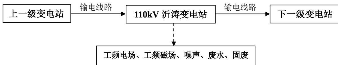
图 1 沭阳 110kV 沂涛变电站扩建#1 主变工程工艺流程及产污环节示意图
