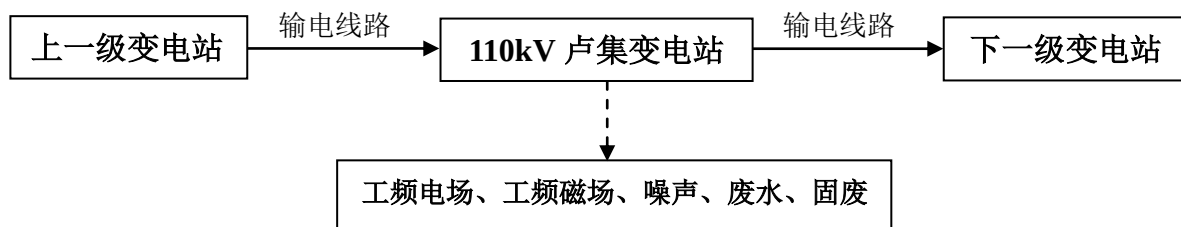
图 1 泗阳 110kV 卢集变电站扩建#1 主变工程工艺流程及产污环节示意图
