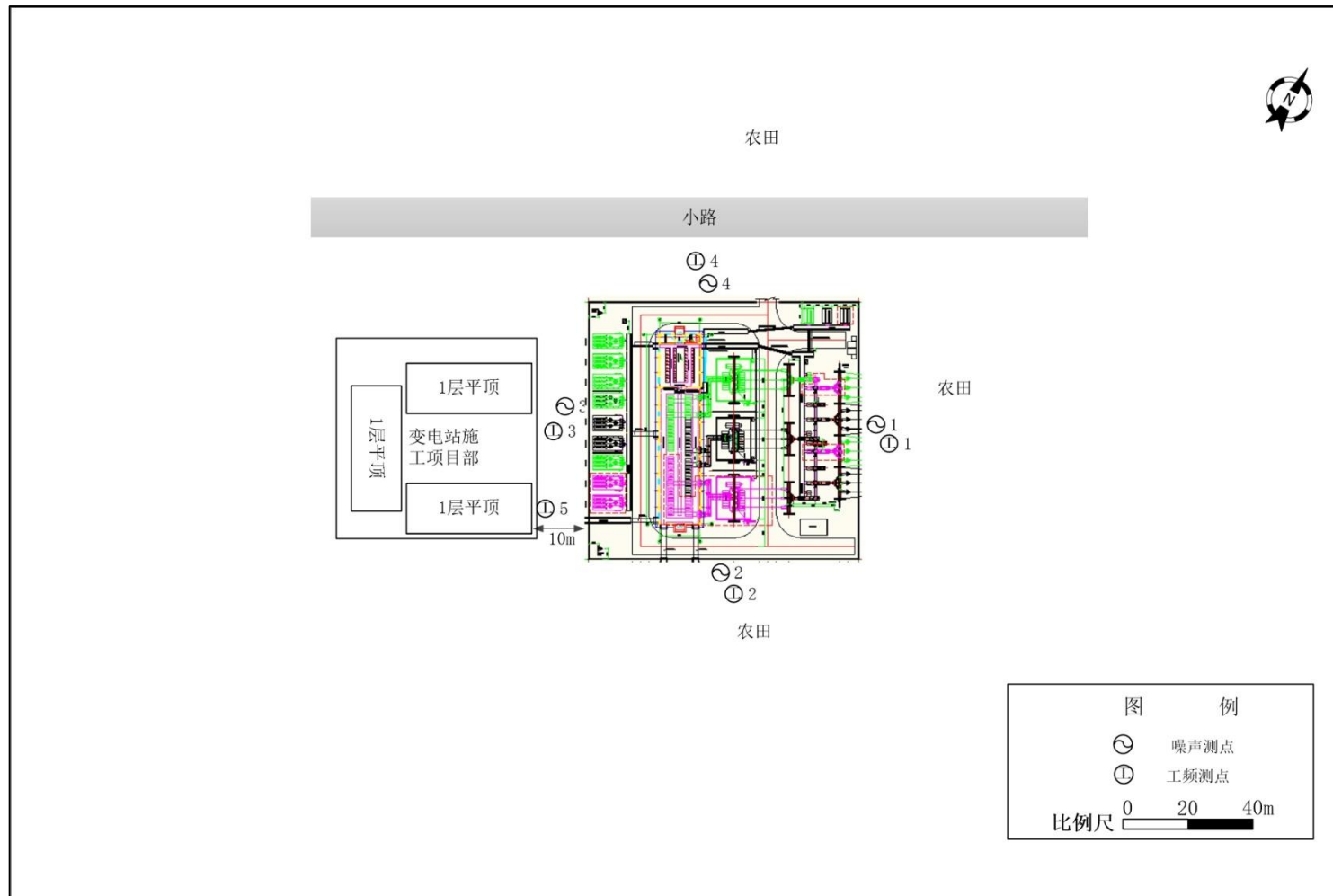
附图 2 110kV 卢集变电站监测点位及周围环境示意图
