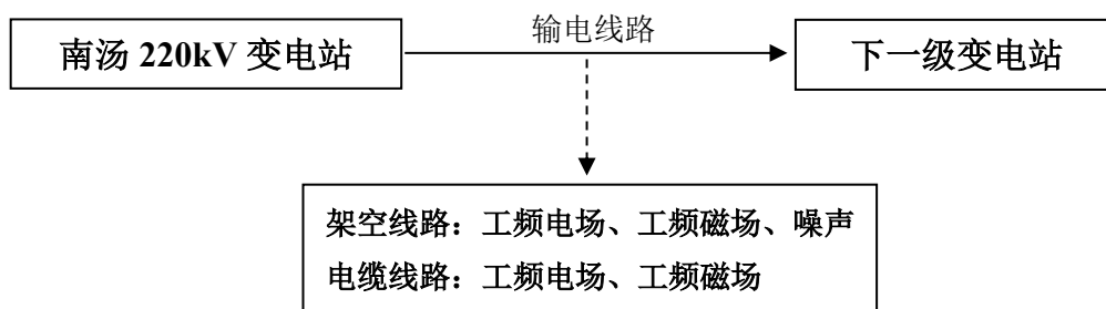
图 1 江苏常州南汤 220kV 变电站 110kV 送出工程工艺流程及产污环节示意图
