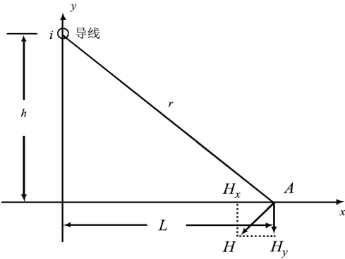
图 3.2-4 磁场向量图
