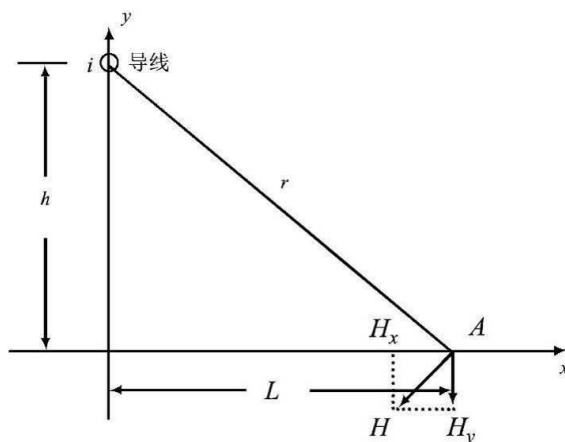
图 3.1-4 磁场向量图
