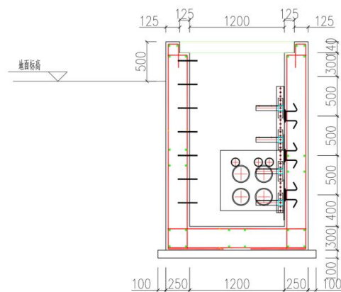
图 1.1-4 电缆井 DL1 土建断面图
