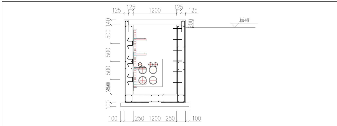
图 1.1-5 电缆井 DL2 土建断面图
