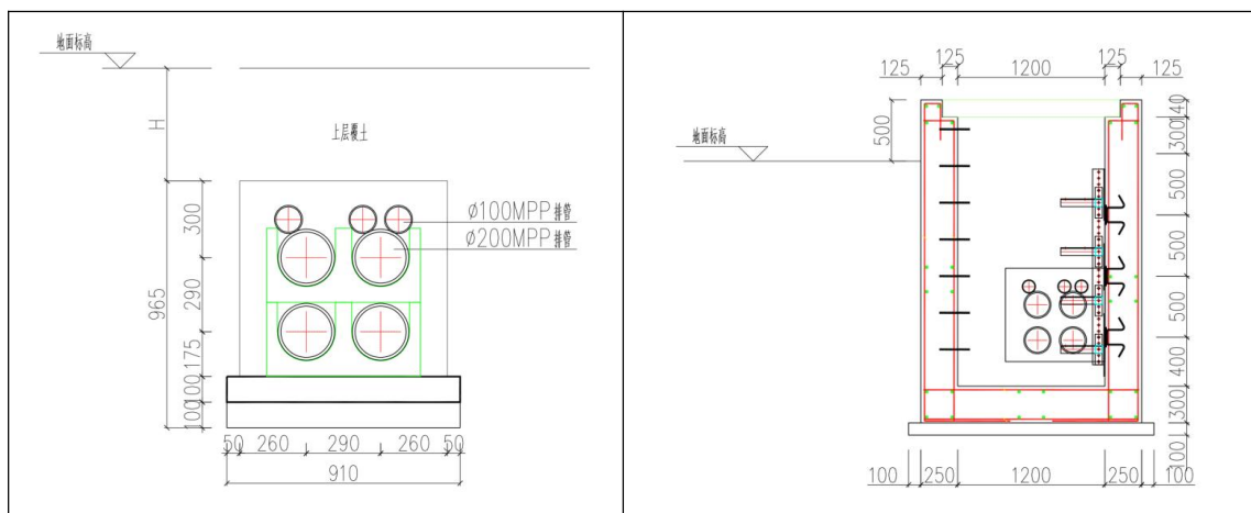
图 1.1-3 电缆排管断面图
