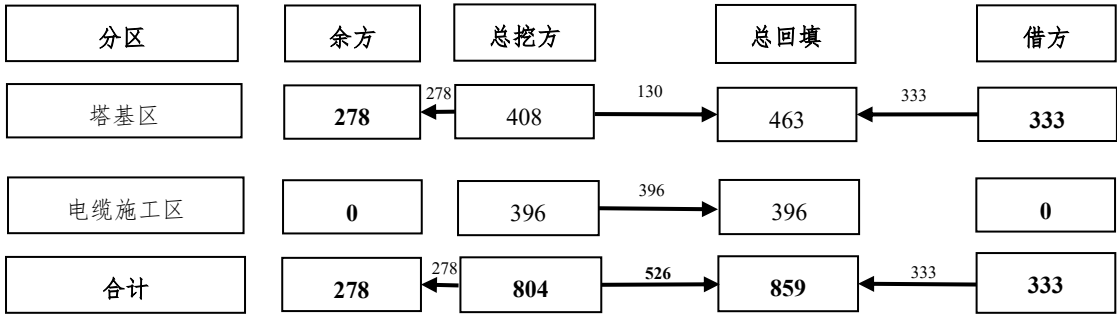
图 1.1-6 土石方平衡流向框图 单位：m 3
