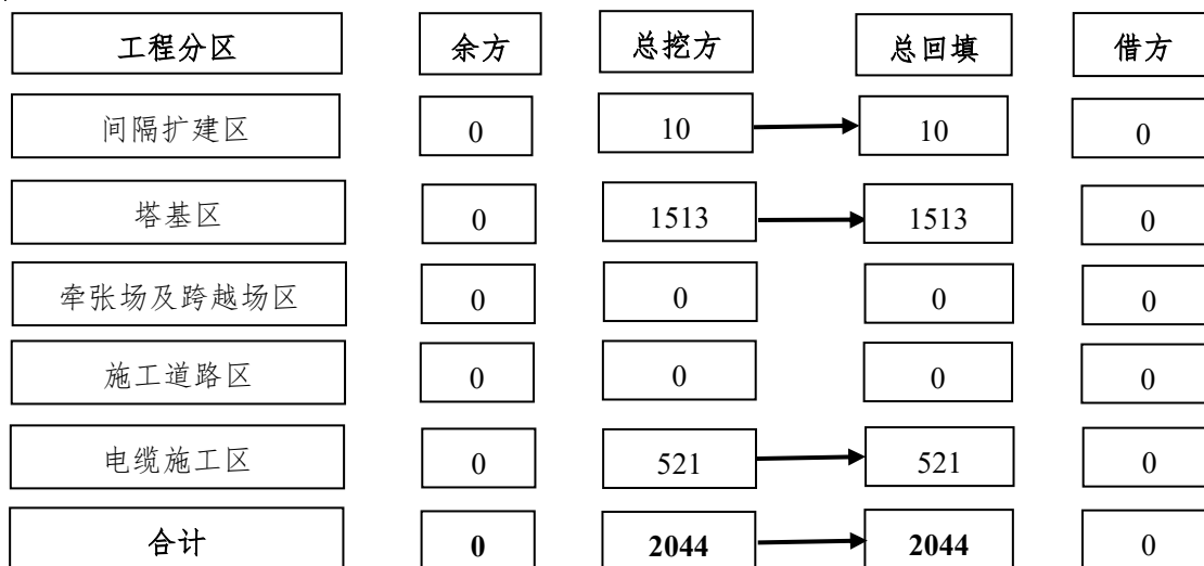
图 1.1-9 土石方平衡流向框图 单位：m 3
