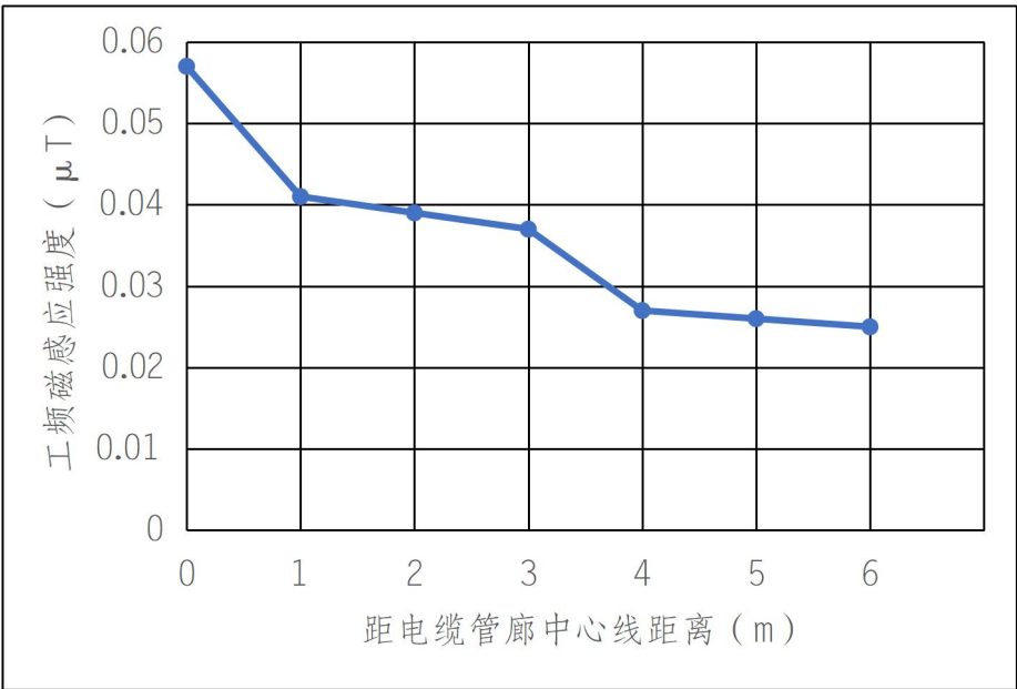
图 7-4 110kV 临红 893 线/110kV 东红 8MC 线电缆线路断面监测处工频磁感应强度趋势图
