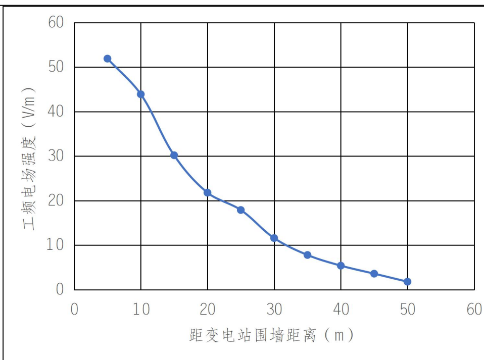
图 7-1 红星 110kV 变电站断面监测处工频电场强度趋势图
