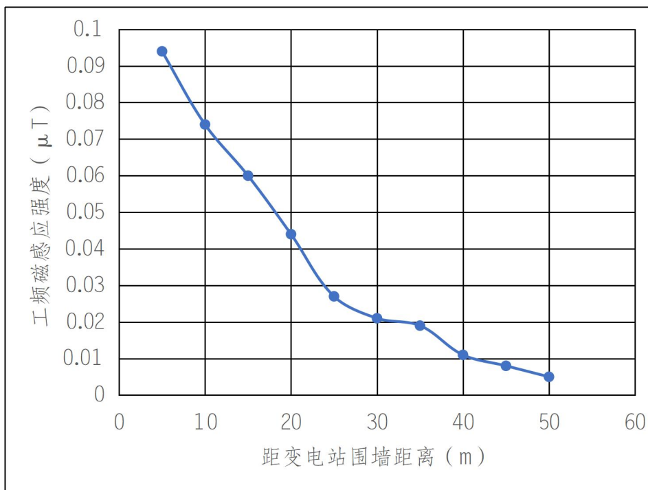
图 7-2 红星 110kV 变电站断面监测处工频磁感应强度趋势图
