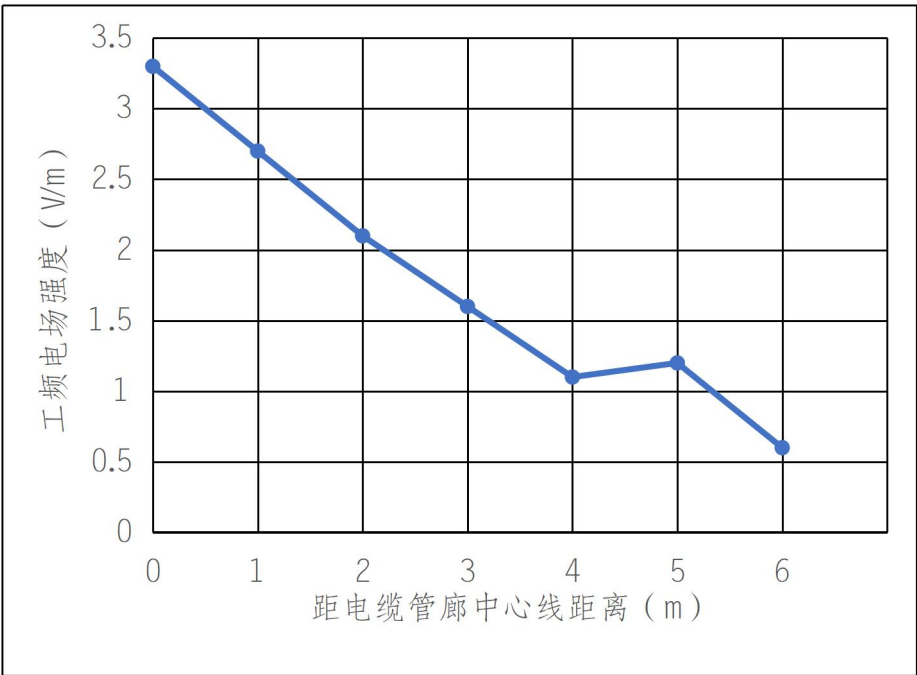
图 7-3 110kV 临红 893 线/110kV 东红 8MC 线电缆线路断面监测处工频电场强度趋势图
