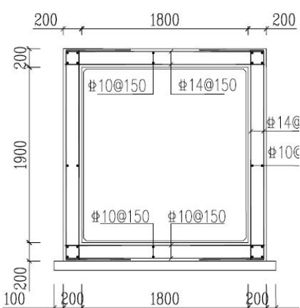
图 1.1-7 余缆井断面图
