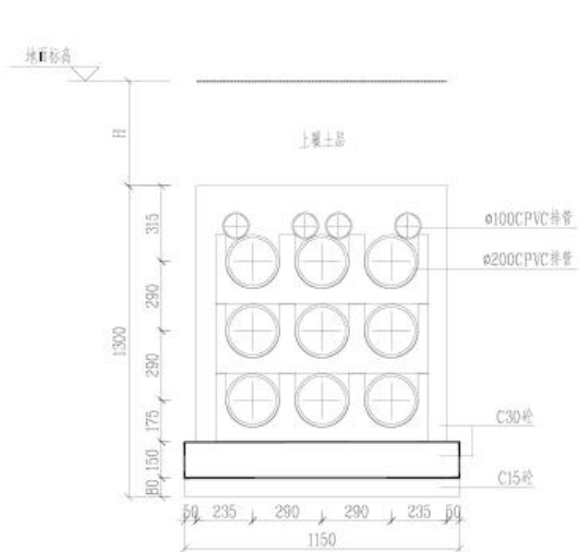
图 1.1-4 电缆排管断面图
