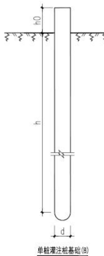
图 1.1-3 塔基基础示意图
