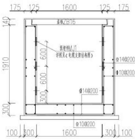
图 1.1-6 转角井断面图
