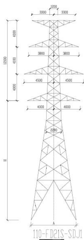
图 1.1-2 塔基型号示意图
