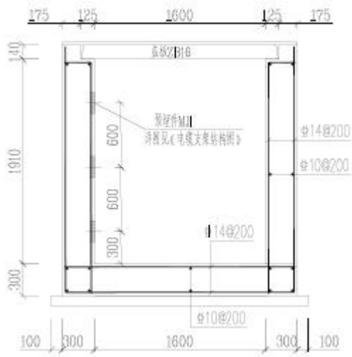
图 1.1-5 直线井断面图
