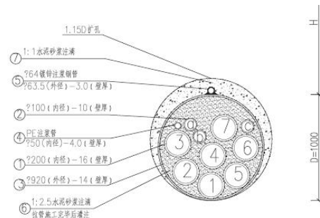
图 1.1-5 电缆拉管断面图
