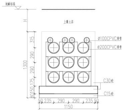
图 1.1-4 电缆排管断面图
