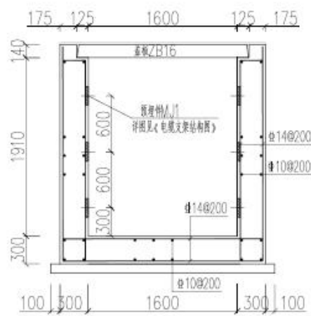
图 1.1-7 转角井断面图
