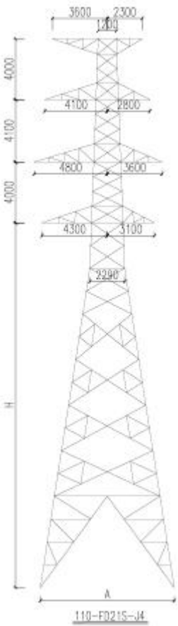
图 1.1-2 塔基型号示意图
