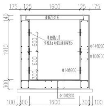
图 1.1-6 直线井断面图
