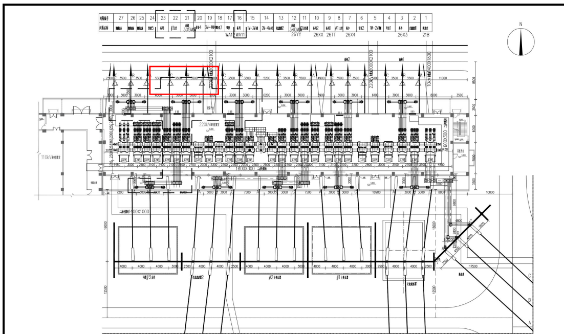
图 1.1-1 少游±200 千伏换流站 220 千伏间隔扩建工程总平面布置图（红框内为扩建间隔）
