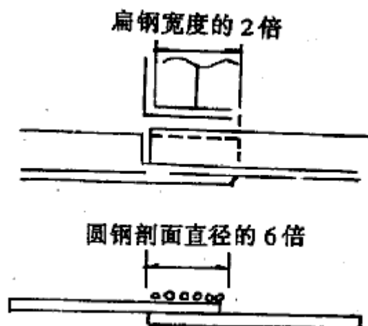
图 3 焊接时搭接长度要求
