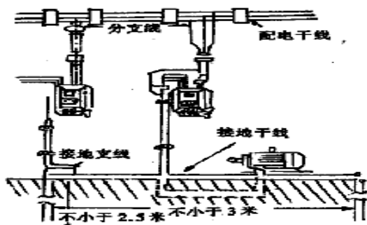
图 2 接地线与接地体示意图
