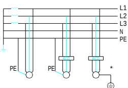
三相 (三线, 三极) TN-S
