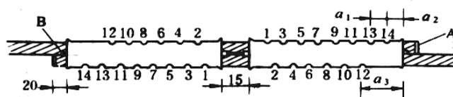
(III) LGJ-240 钢芯铝绞线
