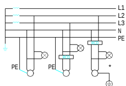
单相 (单极或双极) TN-S
