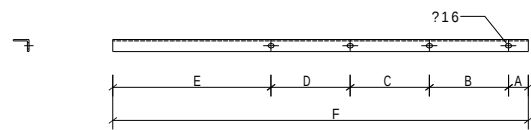
四眼角钢制造尺寸（毫米）
