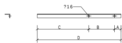
两眼角钢制造尺寸（毫米）
