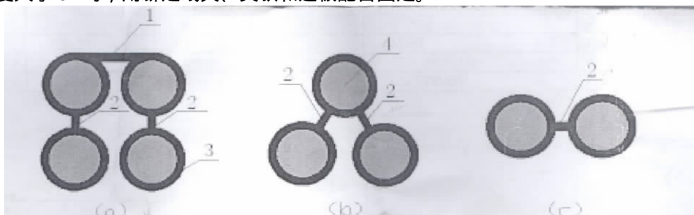
图 9.9.1.4 平行集束导线结构形状断面示意图
