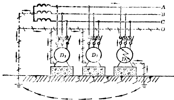
图 2-12 同一供电系统中同时采用接地、接零两种保护方式时的危险性
