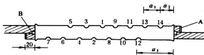
(II) LGJ-35 钢芯铝绞线
