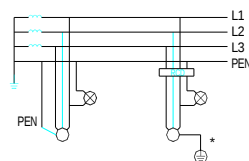
三相 (四线, 三极或四极) TT
