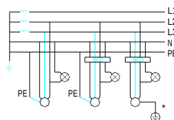
三相 (四线, 三极或四极) TN-S
