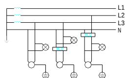
单相 (单极或双极) TT
