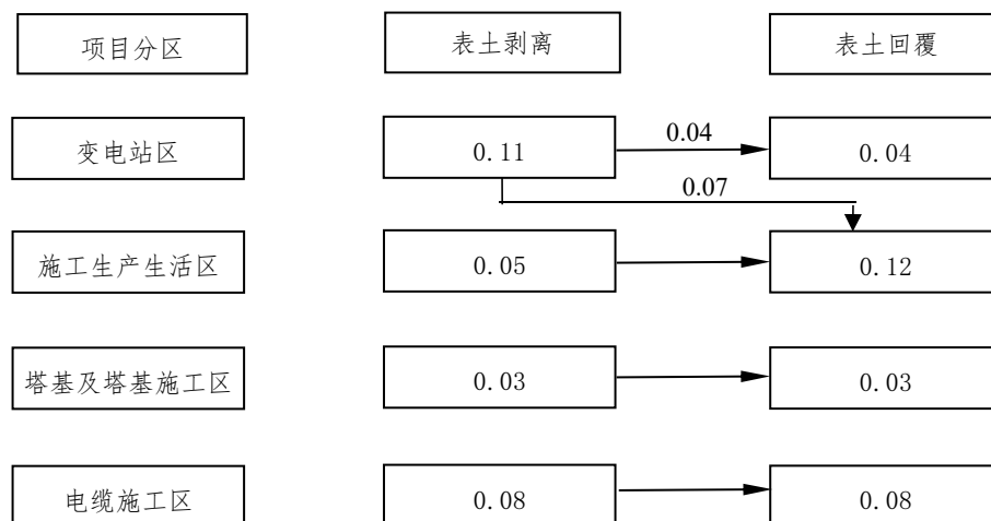
图 1.1-10 表土平衡流向框图 单位：万 \text{m}^3
