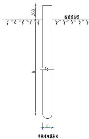
图 1.1-5 塔基基础示意图
