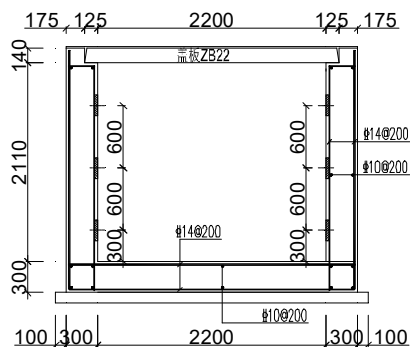
图 1.1-8 接头井断面图
