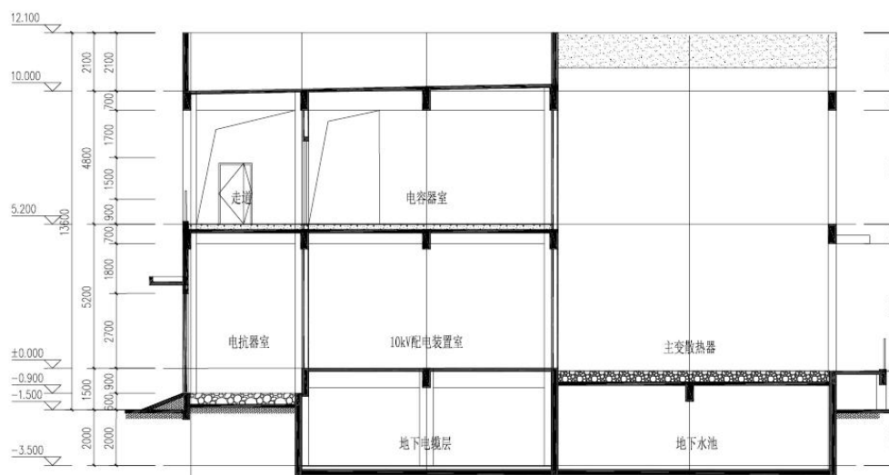
图 1.1-3 配电装置楼剖面图
