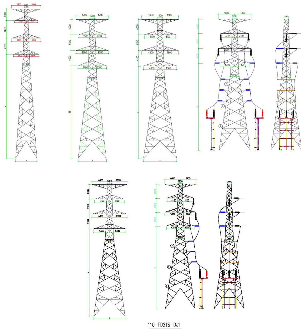
图 1.1-4 塔基型号示意图
