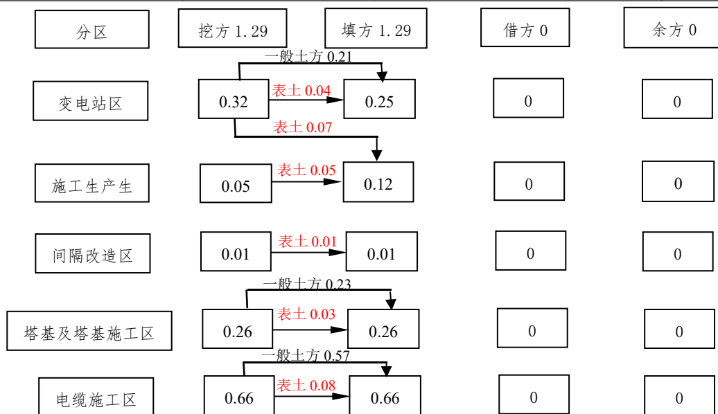
图 1.1-7 土石方平衡框图 单位: 万 m 3
