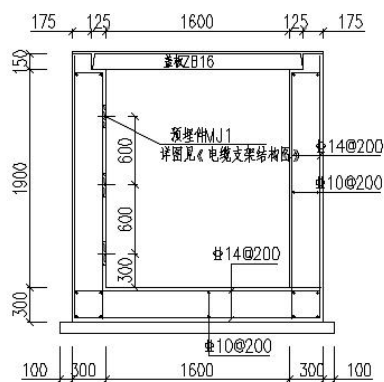
图 1.1-9 三通井断面图
