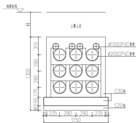
图 1.1-6 电缆排管断面图
