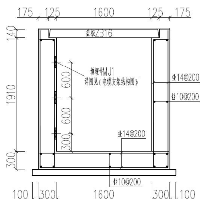
图 1.1-7 直线、转角井断面图
